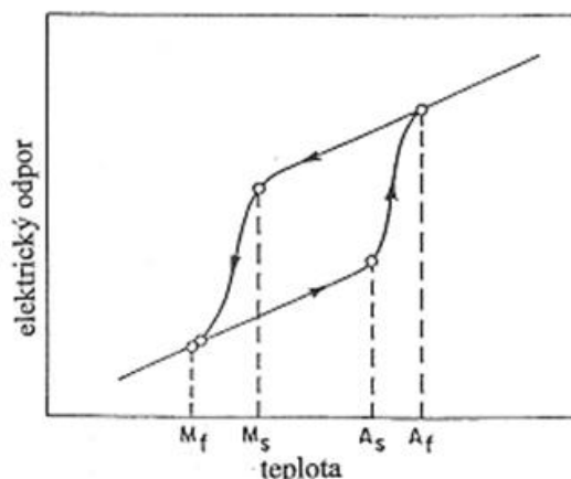
Obrázek 2.2.1 a) Teplotní závislost elektrického odporu slitiny s tvarovou pamětí [2]
