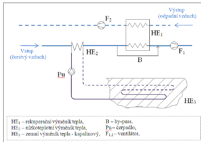
Obr. 2: Větrací systém 1 - schéma
