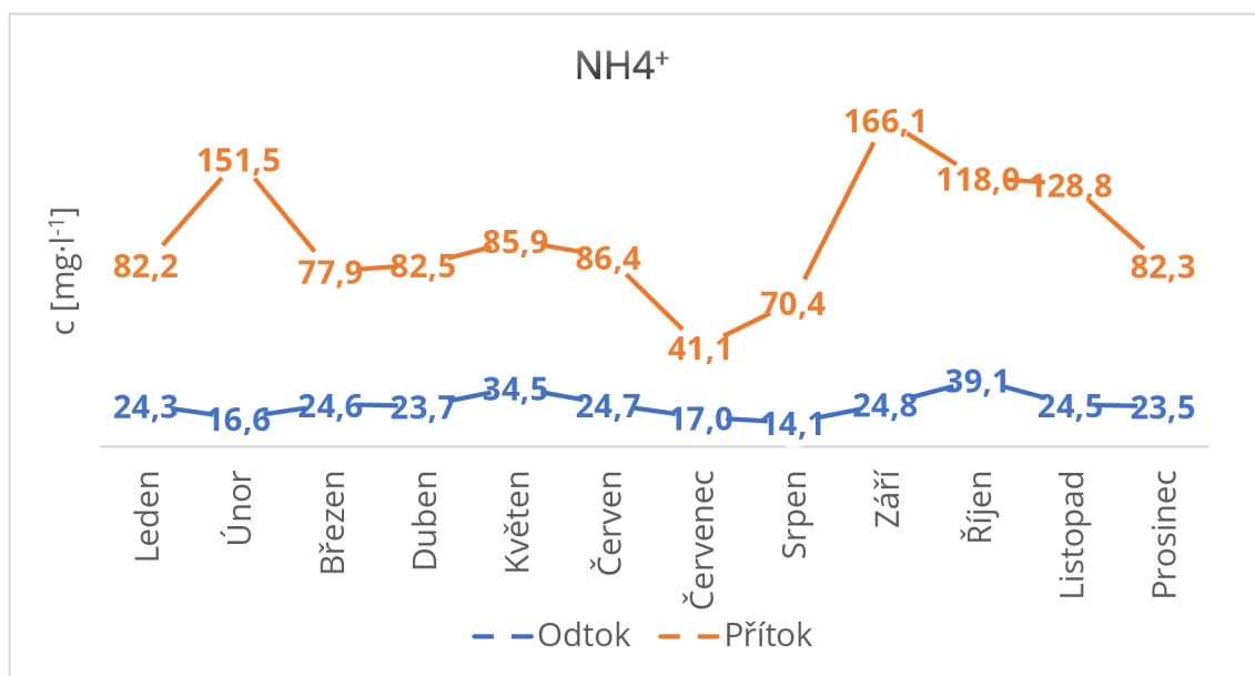
Graf 8 Koncentrace přítoku a odtoku NH + (ČOV Závada)
