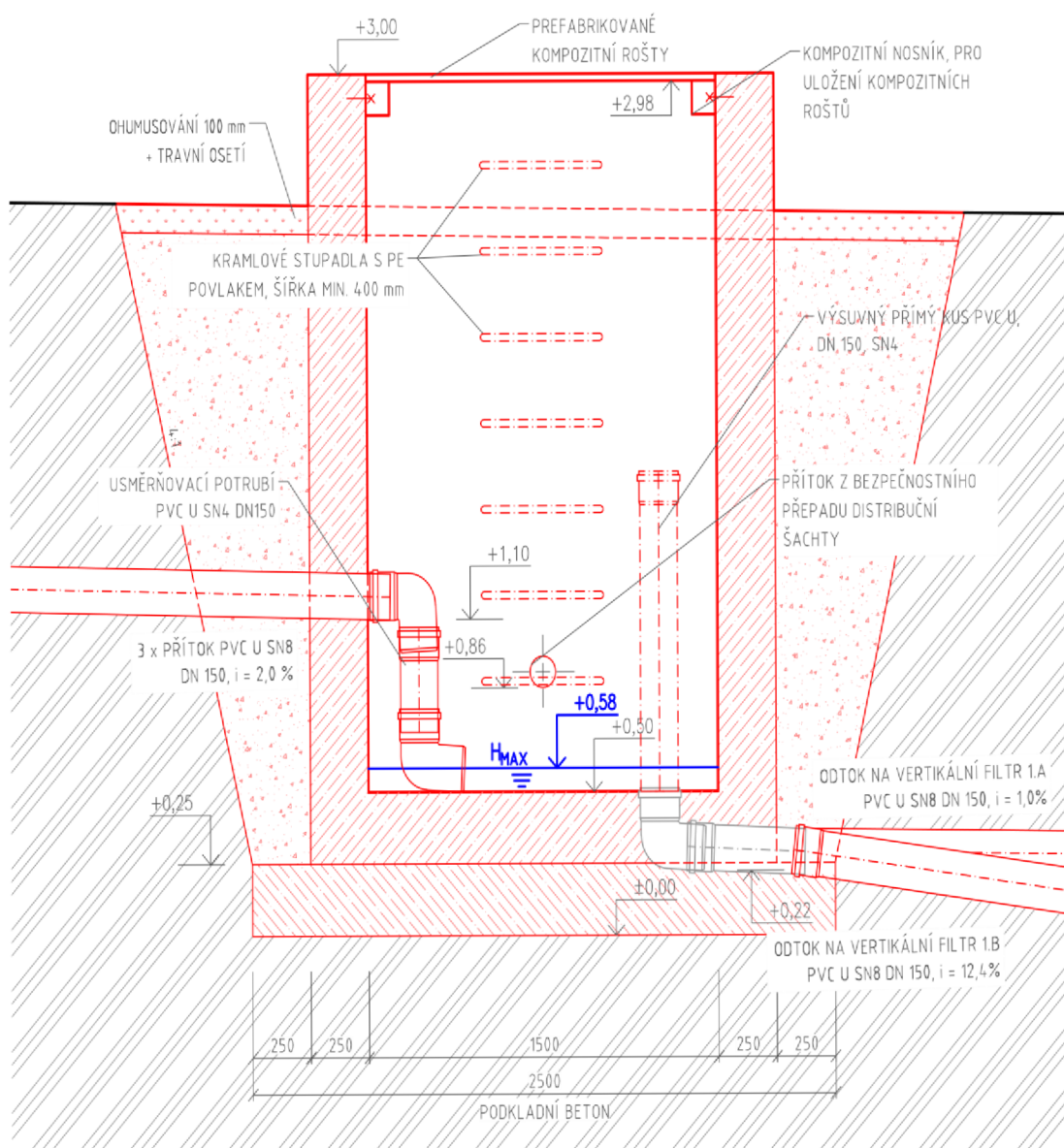
Obrázek 7 Řez rozdělovací šachtou
