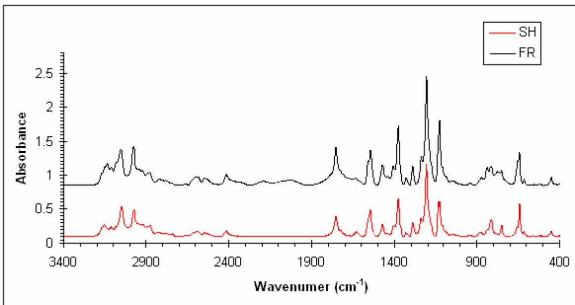
Fig. 37 The measured IR spectrum of NC 1 H-Cl (FR) (Nujol, KBr) \nu (cm -1 ): 451 (vw), 615 (vw), 642 (w), 654 (w), 750 (vw), 779 (vw), 810 (vw), 820 (vw), 839 (vw), 872 (vw), 1107 (vw), 1124 (m), 1207 (vs), 1238 (w), 1290 (vw), 1329 (vw), 1377 (m), 1408 (vw), 1441 (vw), 1472 (vw), 1545 (w), 1558 (w), 1632 (vw), 1753 (w), 2021 (vw), 2195 (vw), 2417 (vw), 2548 (vw), 2588 (vw), 2820 (vw), 2876 (vw), 2920 (vw), 2943 (vw), 2978 (w), 3055 (w), 3113 (vw), 3136 (W), 3171 (vw). The measured IR spectrum of NC 1 H-C (SH) (Nujol, KBr) \nu (cm -1 ): 401 (vw), 449 (vw), 615 (vw), 642 (m), 656 (vw), 750 (vw), 812 (w), 841 (vw), 874 (vw), 885 (vw), 1124 (m), 1132 (m), 1207 (vs), 1240 (w), 1290 (w), 1329 (vw), 1377 (m), 1406 (vw), 1441 (vw), 1474 (vw), 1547 (w), 1630 (vw), 1753 (w), 2417 (vw), 2548 (vw), 2588 (vw), 2876 (vw), 2920 (vw), 2976 (w), 3051 (m), 3113 (vw), 3154 (vw)
