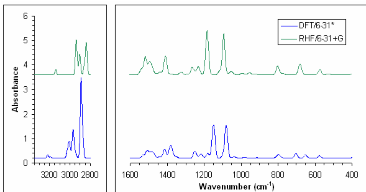
Fig. 34 Predicted IR spectra of \text{NC}_1\text{H-Cl} with DFT/6-31* \nu ( \text{cm}^{-1} ): 573 (vw), 651 (vw), 677 (vw), 731 (vw), 799 (vw), 914 (vw), 982 (vw), 1037 (vw), 1081 (m), 1152 (m), 1180 (vw), 1217 (vw), 1252 (vw), 1383 (vw), 1415 (vw), 1490 (vw), 1508 (vw), 1532 (vw), 2892 (vs), 2967 (w), 3007 (w), 3219 (vw) and RHF/6-31+G \nu ( \text{cm}^{-1} ): 523 (vw), 571 (vw), 678 (w), 799 (vw), 951 (vw), 992 (vw), 1051 (vw), 1092 (vs), 1182 (vs), 1227 (vw), 1263 (vw), 1322 (vw), 1405 (m), 1437 (vw), 1494 (w), 1517 (m), 2839 (s), 2905 (m), 2939 (s), 3143 (vw)
