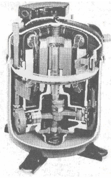
Obr. 8 Řez pístovým kompresorem
