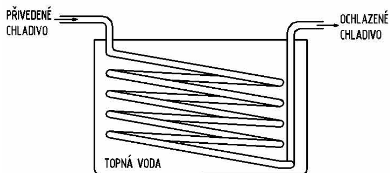
Obr. 13 Trubkový výměník
