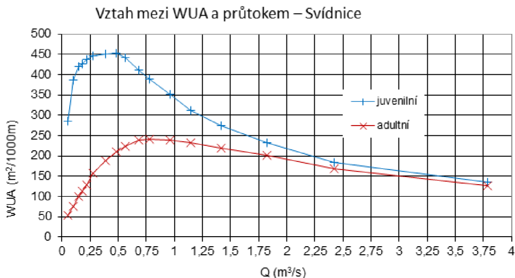
Obrázek č. 2.9 – Vztah mezi WUA a průtokem v rámci studie na Svídnici, a to pro dospělé (adultní) a nedospělé (juvenilní) jedince [59].
