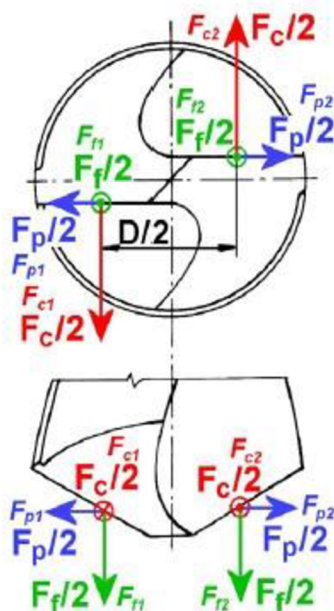
Obr. 25) Rozložení sil při vrtání na standartním šroubovitém vrtáku [13]
