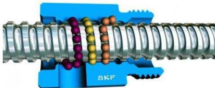
Obr. 18) Řez kuličkovým šroubem od firmy SKF [23]
