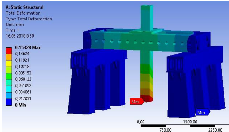
Obr. 52) Deformace příčniku
