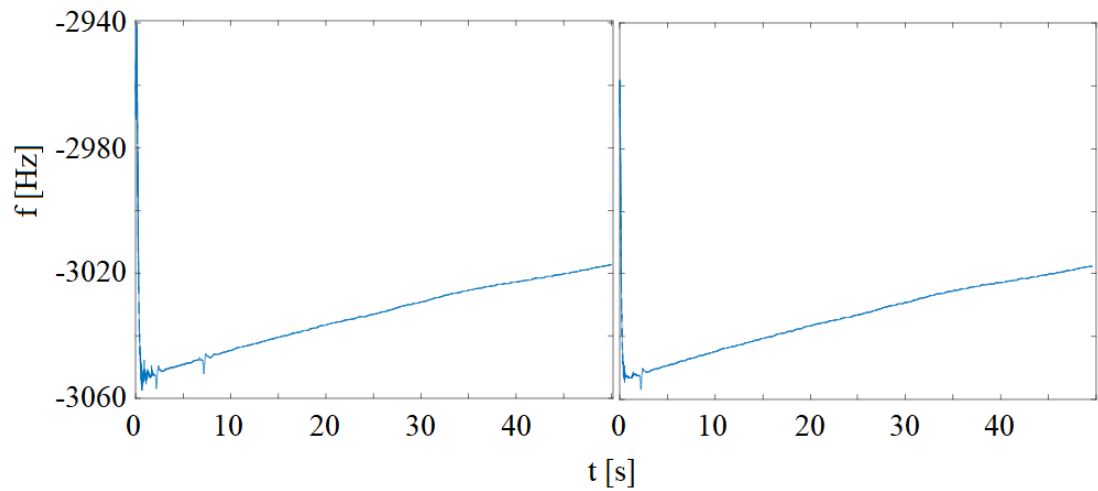
Obr. 4.26 Družice číslo 5, vlevo MATLAB, vpravo FPGA, +90 Hz
