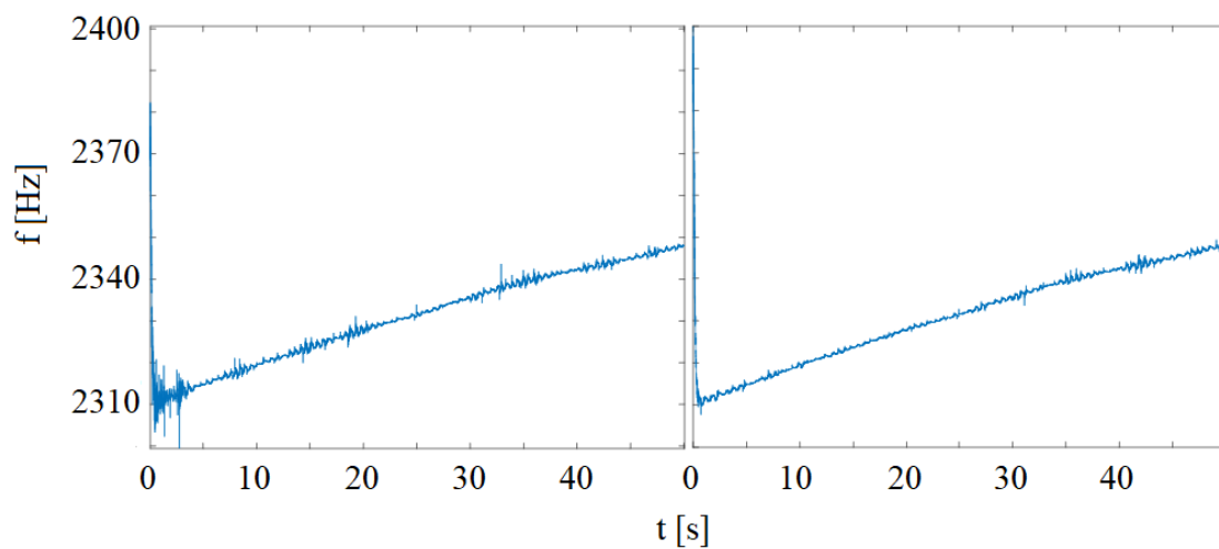
Obr. 4.22 Družice číslo 11, vlevo MATLAB, vpravo FPGA, +90 Hz
