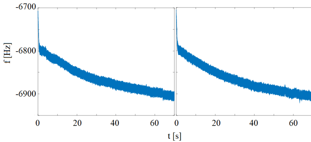
Obr. 4.3 Družice číslo 10, vlevo MATLAB, vpravo FPGA, +90 Hz
