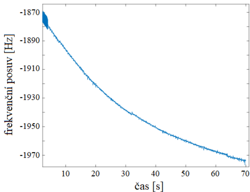
Obr. 2.9 Frekvenční posuv sledovaný Costasovou smyčkou, L1 C/A.
