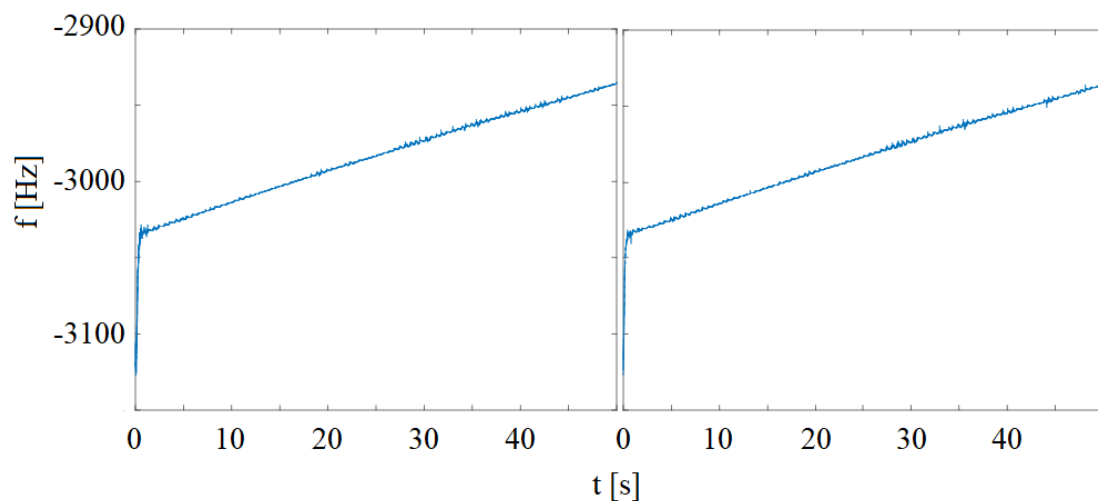
Obr. 4.23 Družice číslo 14, vlevo MATLAB, vpravo FPGA, -90 Hz
