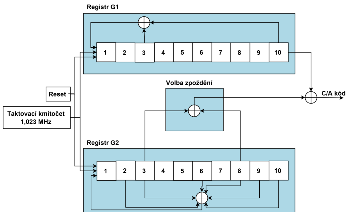
Obr. 1.2 Blokové schéma generátoru C/A kódu.
