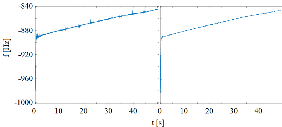
Obr. 4.21 Družice číslo 9, vlevo MATLAB, vpravo FPGA, -90 Hz
