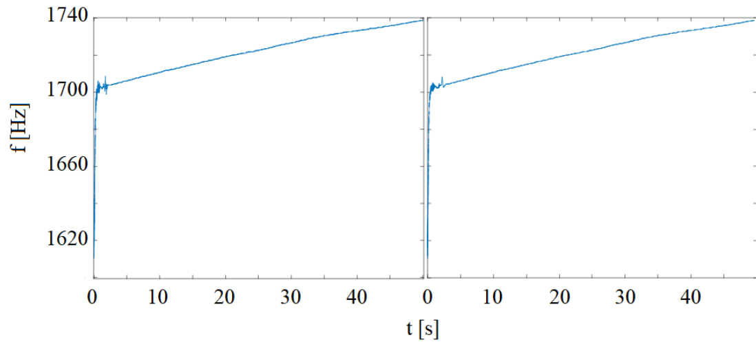
Obr. 4.25 Družice číslo 4, vlevo MATLAB, vpravo FPGA, -90 Hz
