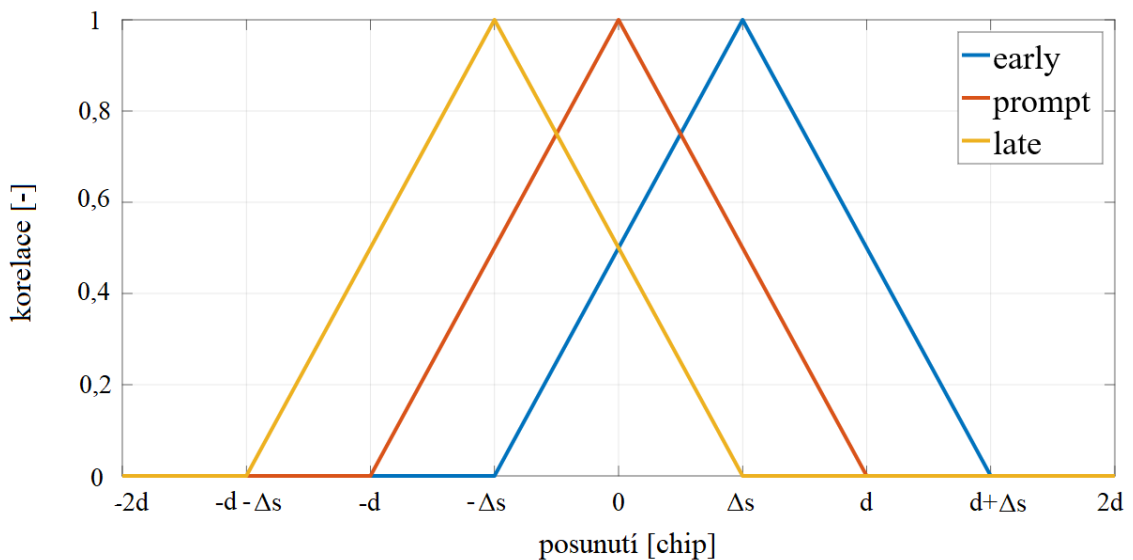
Obr. 2.4 Grafy korelací rozprostíracích sekvencí.
