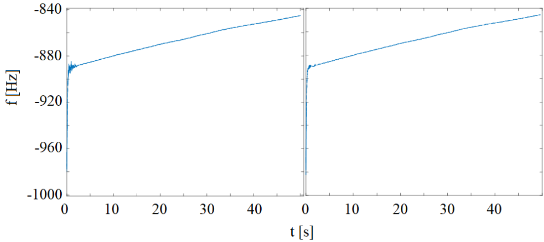
Obr. 4.27 Družice číslo 9, vlevo MATLAB, vpravo FPGA, -90 Hz
