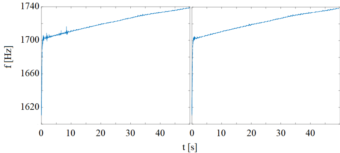
Obr. 4.19 Družice číslo 4, vlevo MATLAB, vpravo FPGA, -90 Hz
