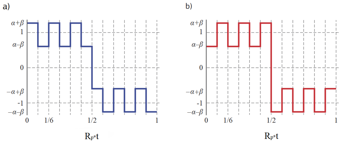
Obr. 1.5 Časové průběhy CBOC subnosných - a) datový signál, b) pilotní signál.
