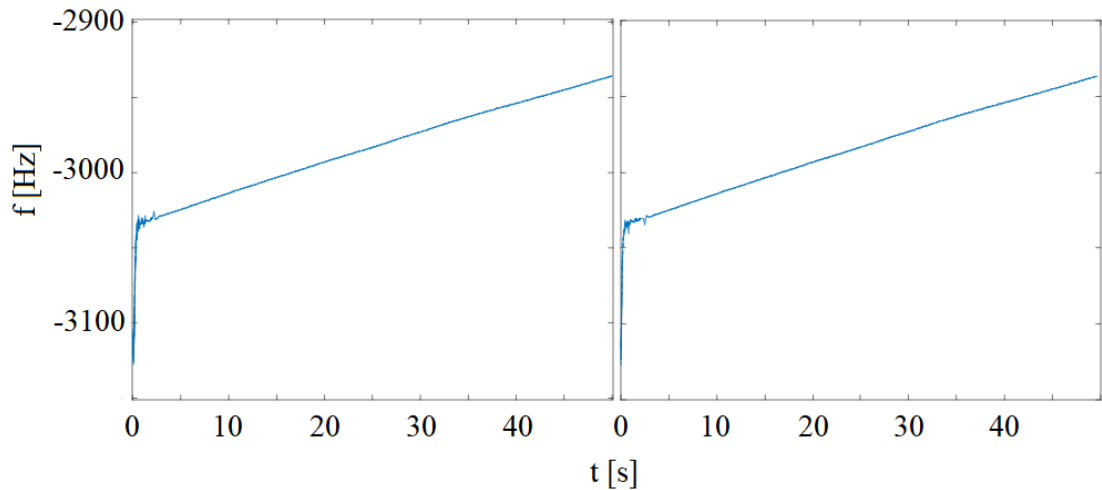
Obr. 4.29 Družice číslo 14, vlevo MATLAB, vpravo FPGA, -90 Hz
