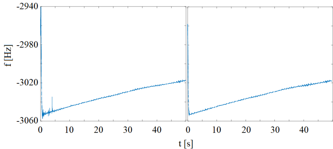
Obr. 4.20 Družice číslo 5, vlevo MATLAB, vpravo FPGA, +90 Hz
