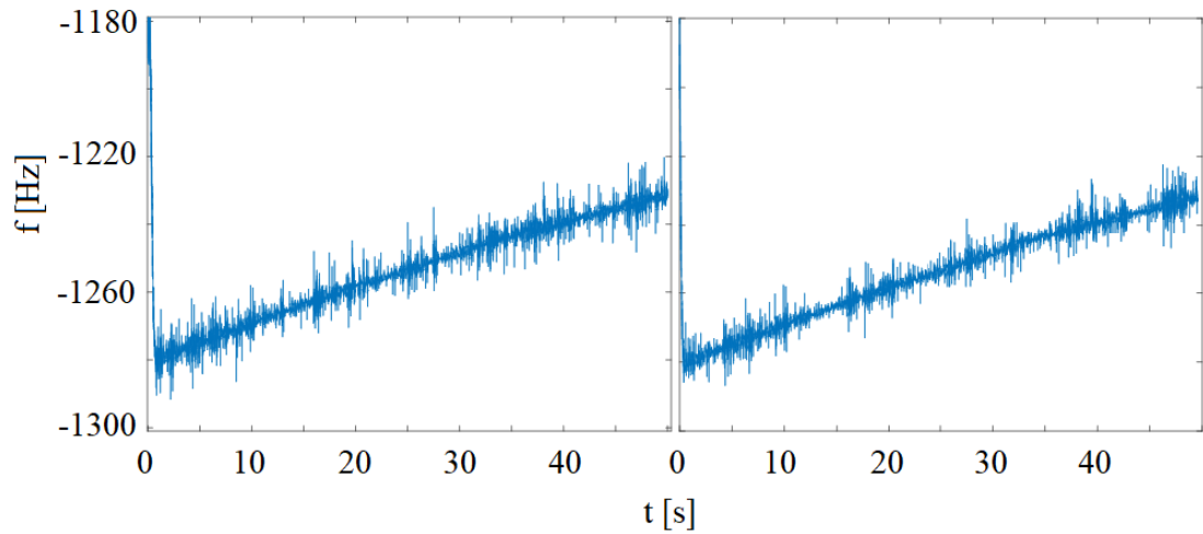
Obr. 4.24 Družice číslo 21, vlevo MATLAB, vpravo FPGA, +90 Hz
