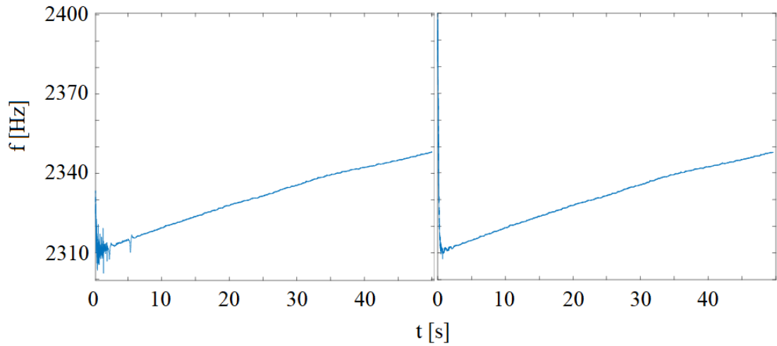
Obr. 4.28 Družice číslo 11, vlevo MATLAB, vpravo FPGA, +90 Hz
