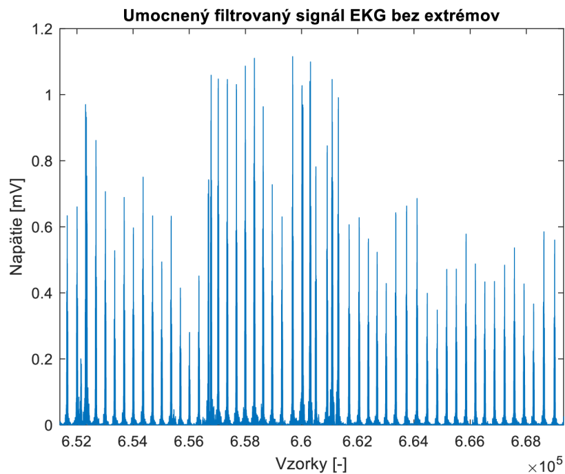
Obr. 5-5 Filtrovaný EKG signál pásmovou priepustou o frekvenciách 10 a 21Hz
