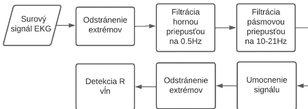
Obr. 5-11 Blokovaná schéma detektoru R vln v signáli EKG
