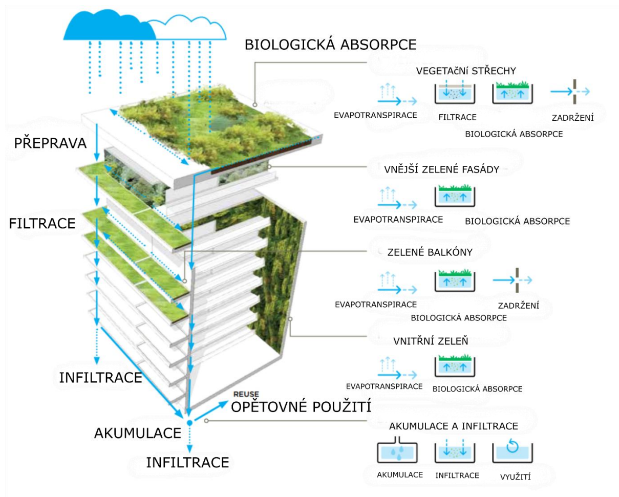
Obrázek 3.5 - Zadržování dešťové vody na budovách [Ramboll, 2016]
