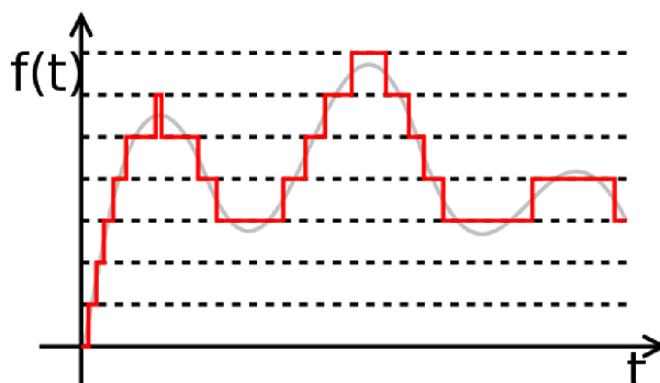
obr. 1-4: Kvantovaný signál
