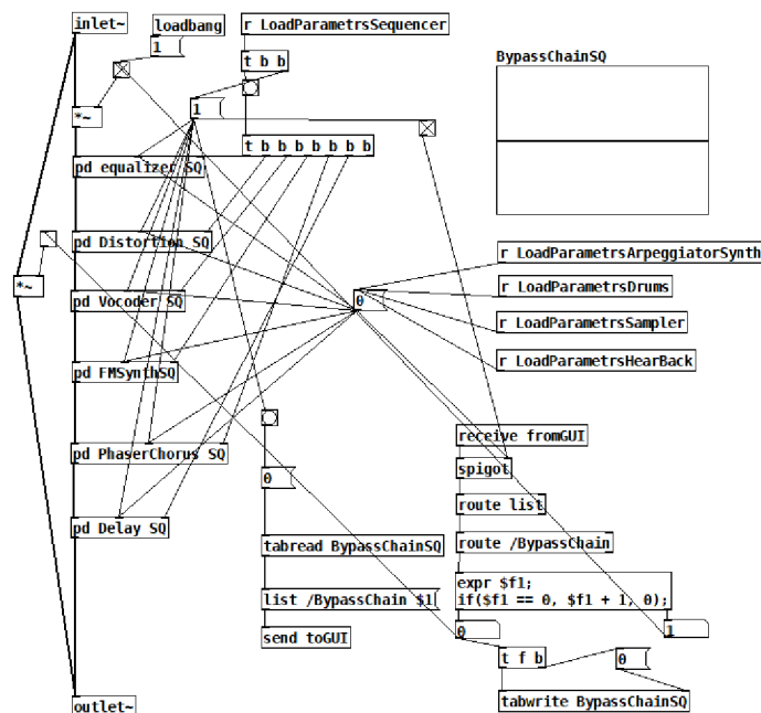
obr. 3-10: Efektová větev pro Sequencer
