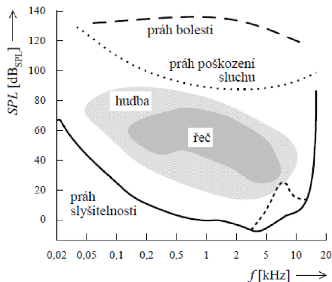
obr. 1-1: Oblast slyšení [6]
