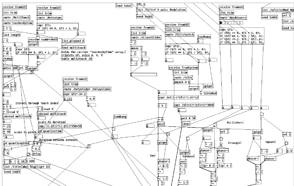
obr. 3-6: Arpeggiator Synth
