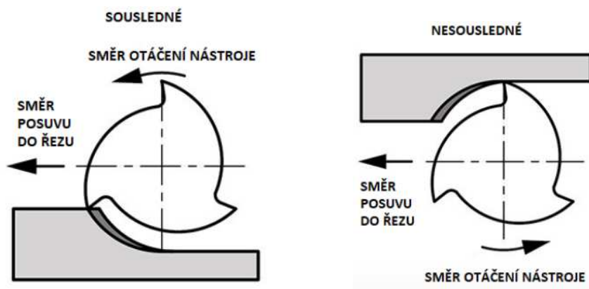
Obrázek 6: Znázornění směru otáčení řezného nástroje [19]
