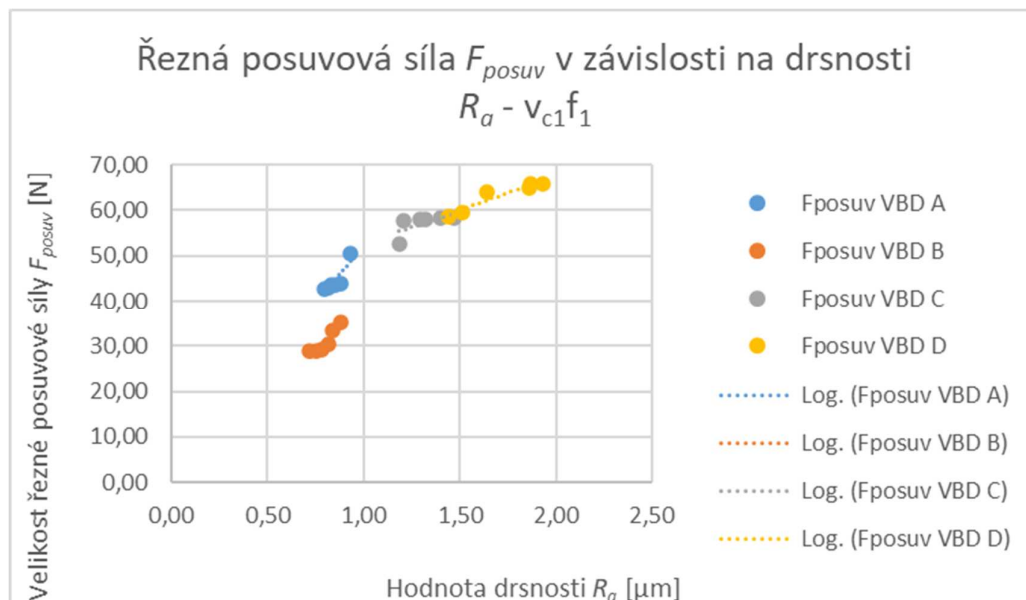
Graf 7: Závislost řezné posuvové síly F_{posuv} na drsnosti povrchu R_a při řezných podmínkách v_{c1}f_1
