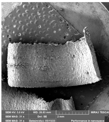
Obrázek 37: Detailní pohled na mikročástice – použit mikroskop SEM
