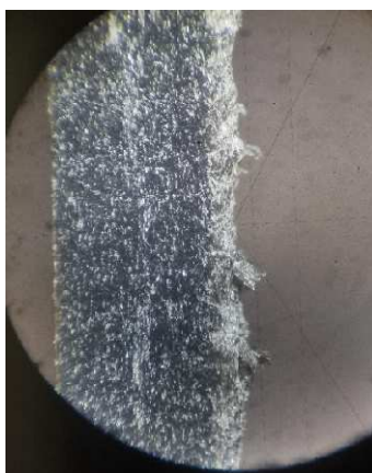
Obrázek 29: Detail delaminace materiálu na dílenském mikroskopu
