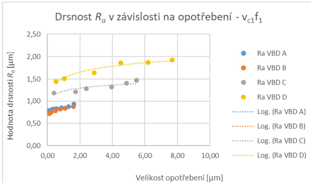
Graf 3: Závislost drsnosti R_a na opotřebení VBD při řezných podmínkách v_{c1}f_1
