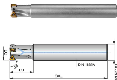
Obrázek 19: Stopková fréza 25A4R034A25-STM10-C [20]
