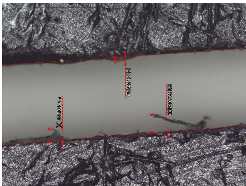
Obrázek 35: Zobrazení delaminace pomocí Keyence – měření B
