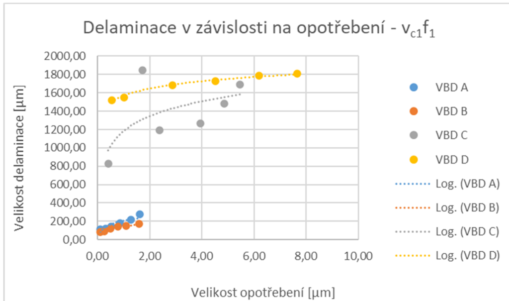
Graf 11: Závislost delaminace na straně vzorků obrobeneho nesousledným frézováním na opotřebení VBD při řezných podmínkách v_{c1}f_1
