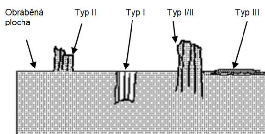
Obrázek 7: Znáornění jednotlivých typů delaminací [23]
