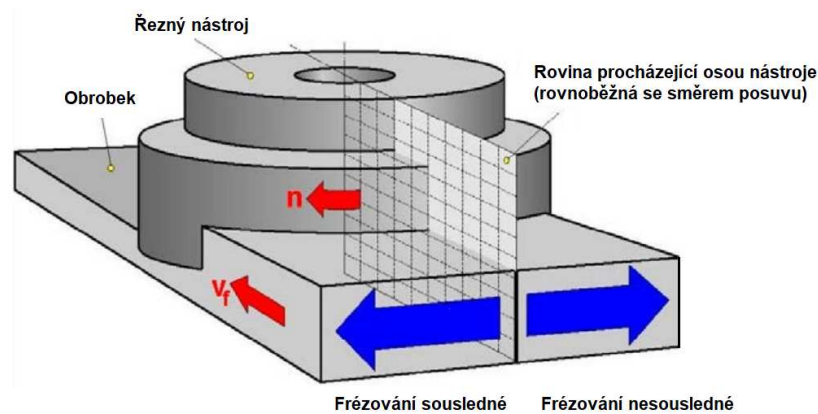
Obrázek 5: Dva druhy frézování – sousledné a nesousledné frézování [35]
