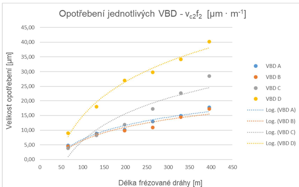
Graf 2: Závislost opořebení jednotlivých VBD při řezných podmínkách v_{c2}f_2
