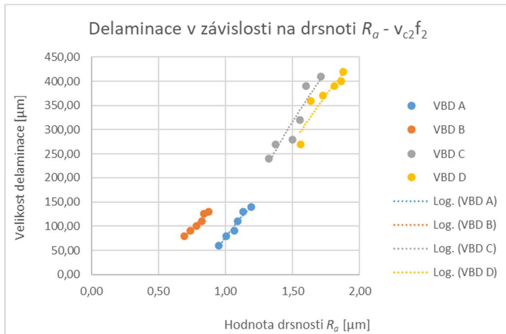
Graf: Závislost delaminace na straně vzorků obrobeneho nesousledným frézováním na drsnosti povrchu R_a při řezných podmínkách v_{c2}f_2
