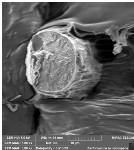
Obrázek 39: Detailní pohled na mikročástice – použit mikroskop SEM
