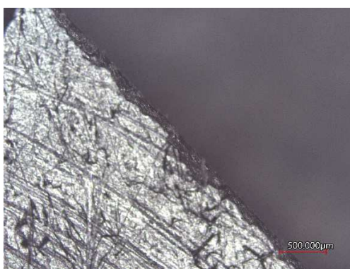
Obrázek 30: Delaminace na Keyence
