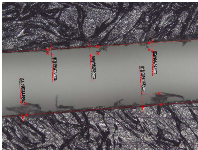
Obrázek 34: Zobrazení delaminace pomocí Keyence – měření A
