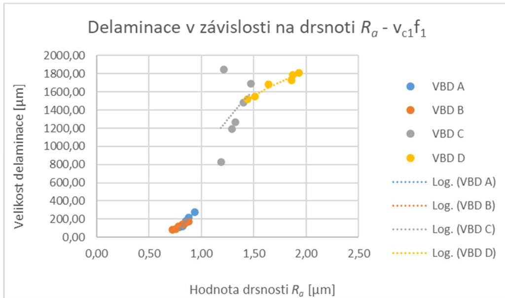
Graf 9: Závislost delaminace na straně vzorků obrobeneho nesousledným frézováním na drsnosti povrchu R_a při řezných podmínkách v_{c1}f_1
