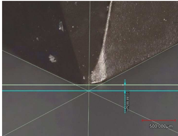
Obrázek 27: Zobrazení opotřebení VBD na mikroskopu od firmy Keyence
