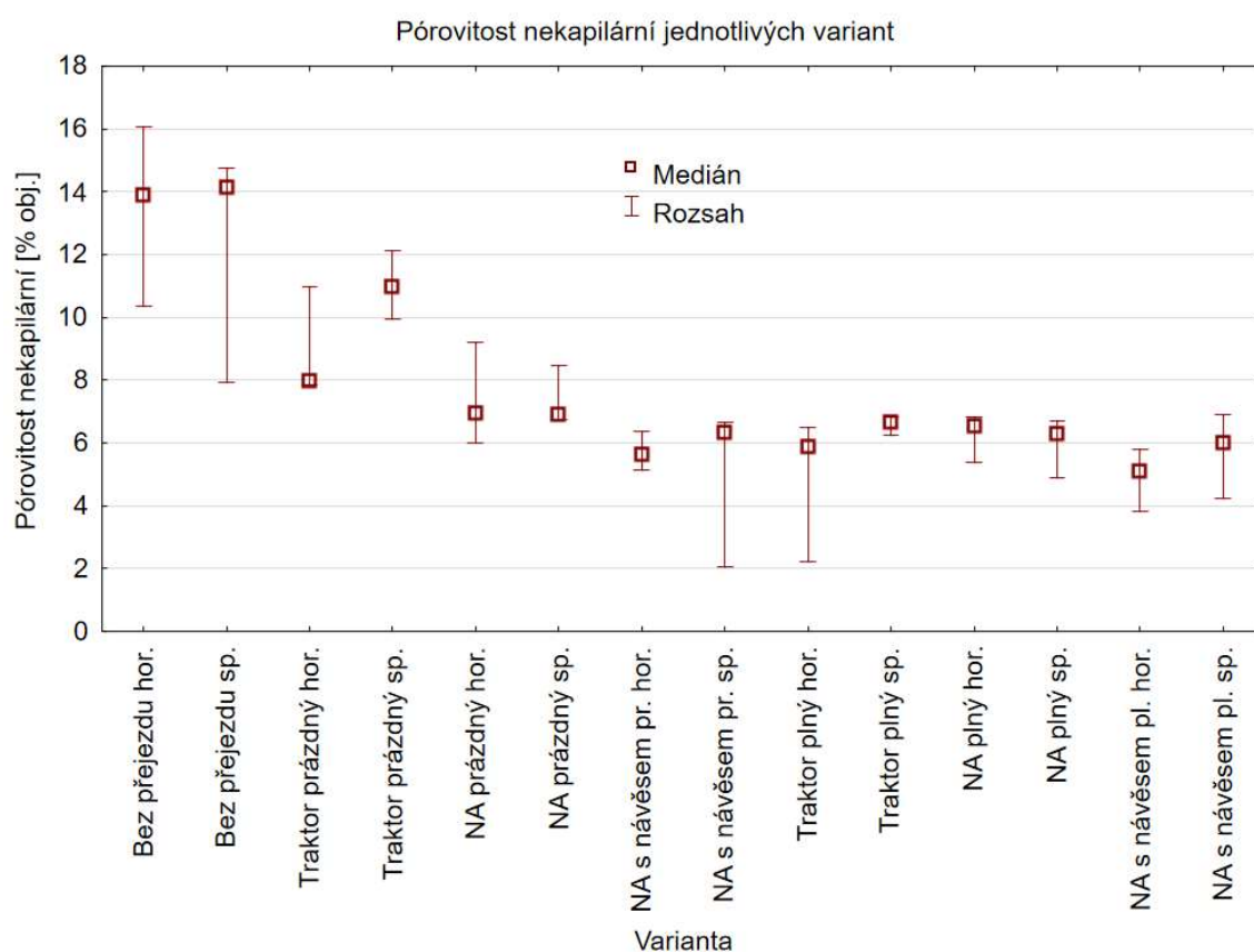
Obrázek 17: Pórovitost nekapilární
