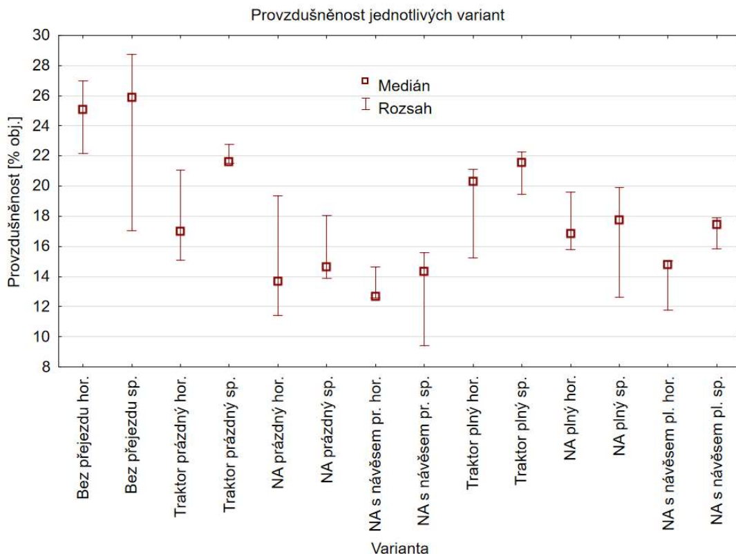
Obrázek 18: Provzdušňenost
