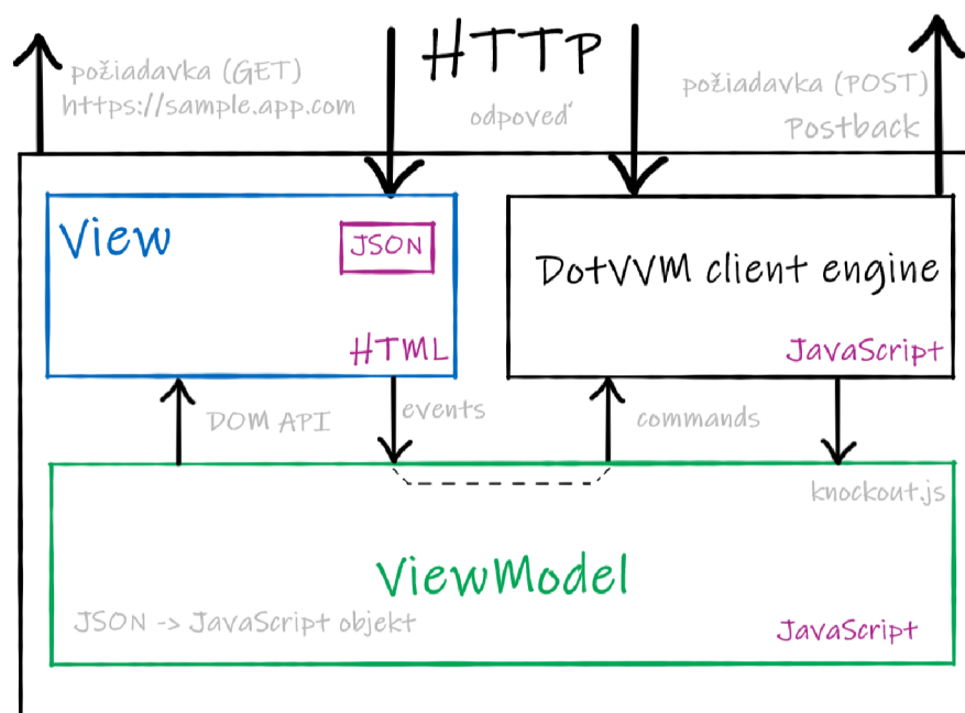
Obr. 6.3: Principiálna schéma fungovania DotVVM v prehliadači
