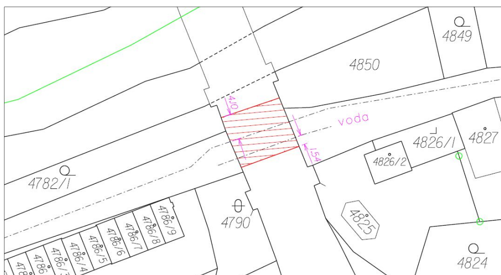
Obr. 13 Výřez z návrhu rozsahu služebnosti inženýrské sítě
