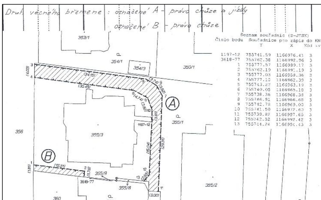
Obr. 25 Výřez z příslušného geometrického plánu
