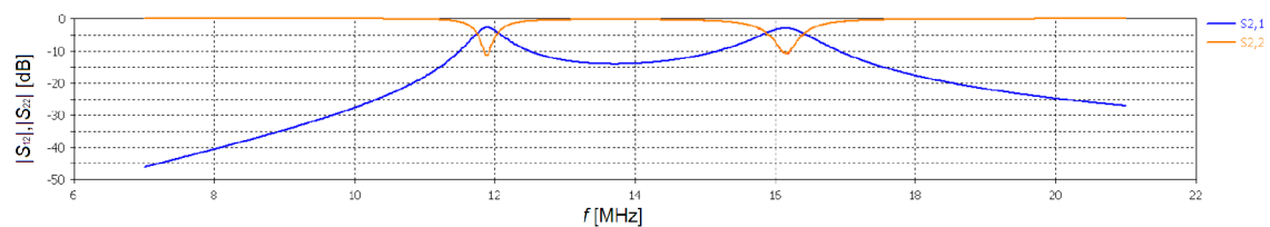
Obr. 4.12: Závislost rozptylových parametrů na frekvenci, vyjádřená v dB; vazba bez překážky
