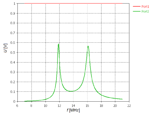
Obr. 4.13: Závislost velikosti napětí na frekvenci; vazba bez překážky
