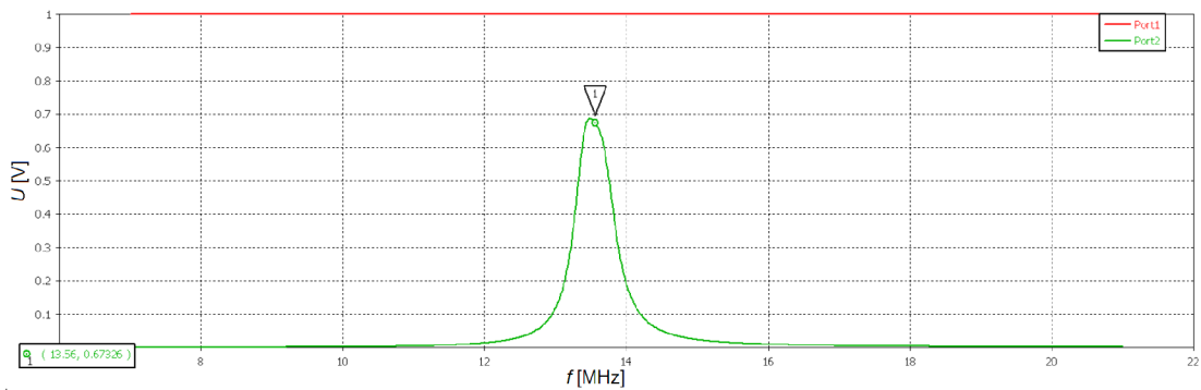
Obr. 4.15: Závislosti velikosti napětí na frekvenci; vazba bez překážky
