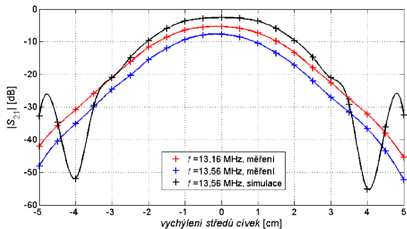
Obr. 7.7: Závislost napěťového útlumu přenosu, vyjádřeného pomocí parametru |S_{21}| , na vychýlování středů cívek doleva (-) a doprava (+), konfigurace S_I - S_II.
