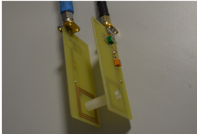
Obr. 7.23: Měření s laditelným přizpůsobovacím obvodem
