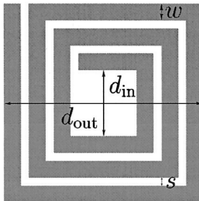
Obr. 2.1: Čtvercová spirálová cívka se zakótovanými rozměry [7]
