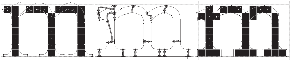
Obrázok 3.9: Obrysy písmena 'm' bez inštrukcií (vľavo) a s inštrukciami (vpravo). Grafická vizualizácia inštrukcií (v strede) Autor: www.microsoft.com
