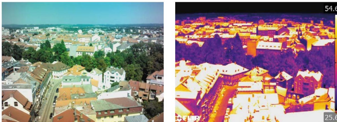
Obrázek 5: Srovnání teplot v části města s vegetací a bez vegetace Zdroj: upraveno z: projekty.pf.jcu.cz
