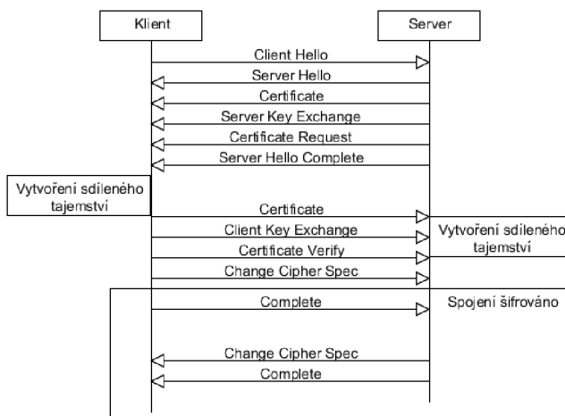
Obr. 3.5 Autentizace EAP-TLS
