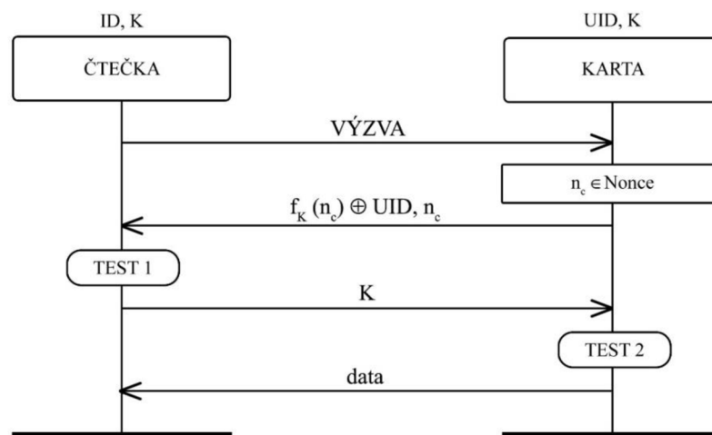
Obr. 4.6 Protokol Weis
