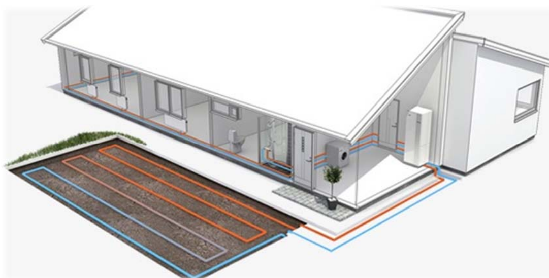
Obr. 17 Plošný kolektor [34]
