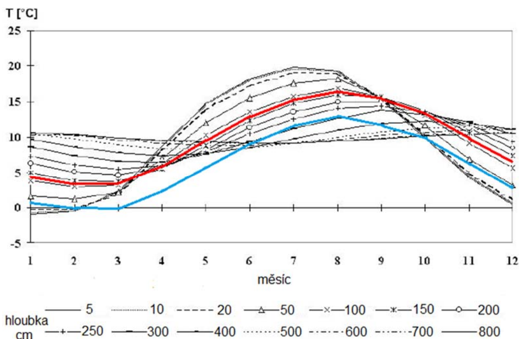
Obr. 33 Průměrný roční průběh teploty zeminy v různých hloubkách (Stropkov; 1984-1997) [25]
