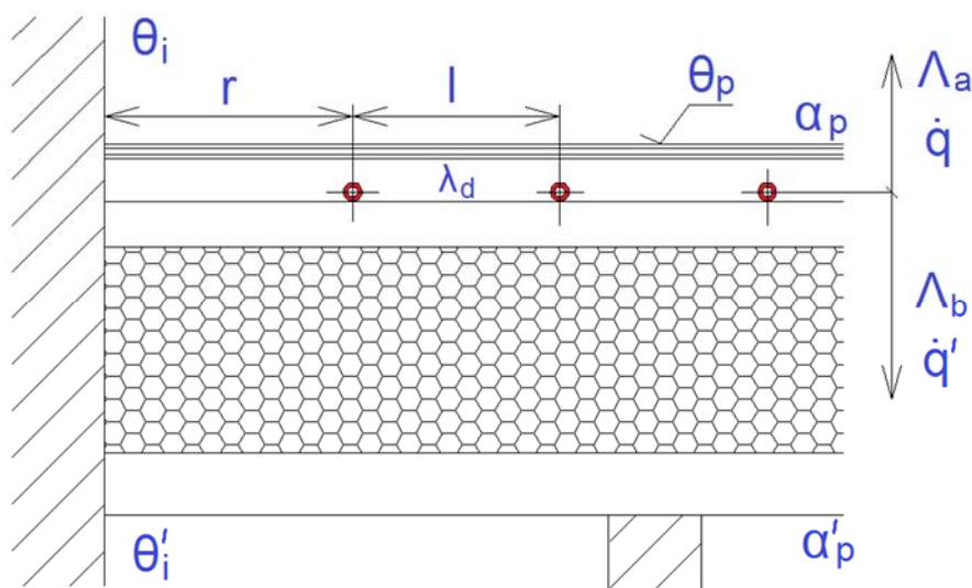
Obr. 30 Řez podlahovou plochou v šicí dílně
