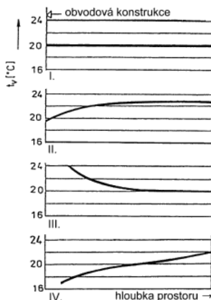
Obr. 3 Horizontální teplotní profil v místnosti u různých forem vytápění; I. – ideální průběh teplot, II. – podlahové vytápění, III. – článekový radiátor, IV. – stropní vytápění [4]
