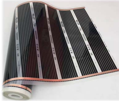
Obr. 16 Elektrická topná fólie [23]
