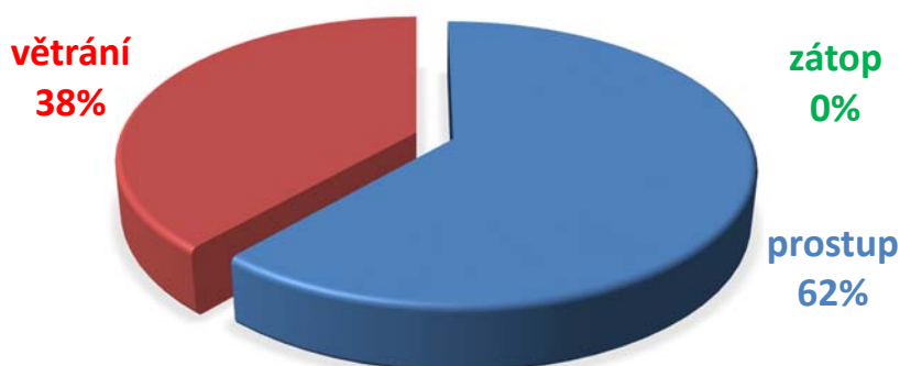
Obr. 27 Graf procentuálního zastoupení jednotlivých složek tepelných ztrát
