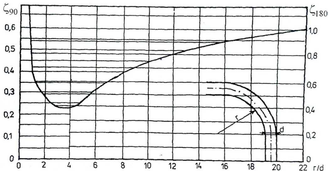
Obr. 31 Součinitel místního odporu pro oblouk 90° a 180° [7]
