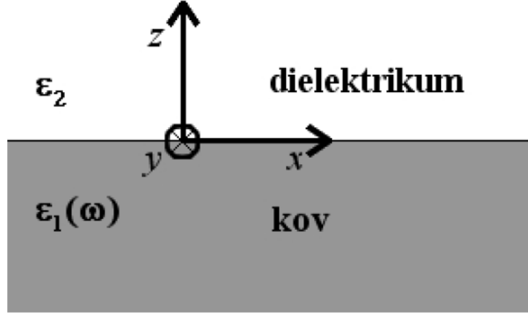
Obrázek 3.1: Rozhraní mezi prostředími. Optické vlastnosti prostředí jsou popsány dielektrickými funkcemi \varepsilon_1 a \varepsilon_2 . Obrázek převzat z [3].
