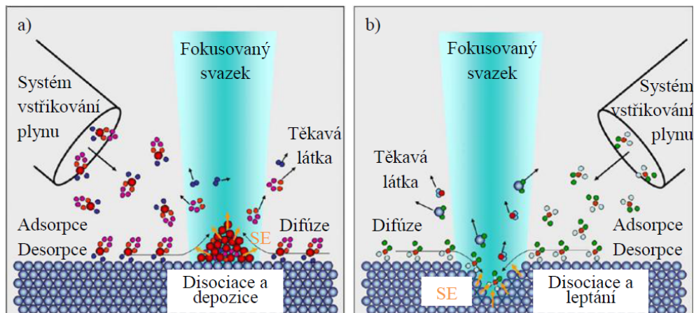
Obrázek 6.1: Zobrazení principu a) depozice a b) leptání indukovaným fokusovaným elektronovým nebo iontovým svazkem (SE – sekundární elektrony). Převzato z [8].
