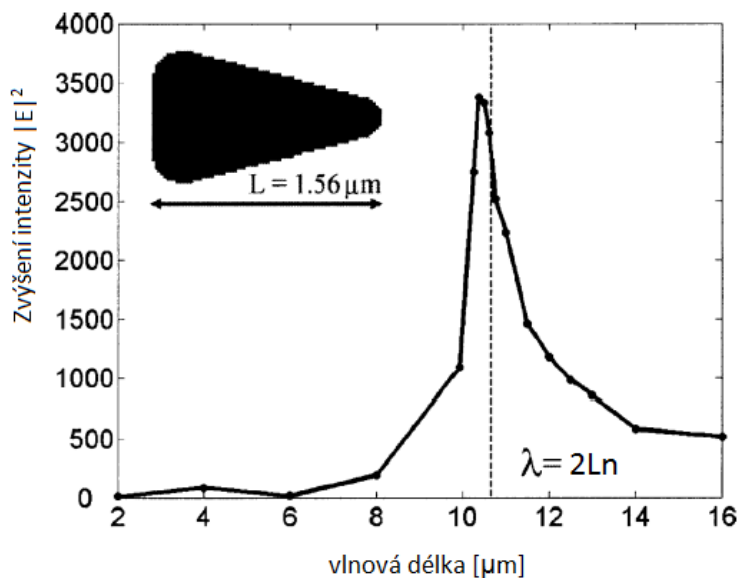
Obrázek 5.1: Graf závislosti zvýšení intenzity elektrického pole |E|^2 vlnové délce, pro antény délky L = 1,56 \mu\text{m} a tloušťky 60 \text{ nm} s vrcholovým úhlem 30^\circ , v poli antén vzdálených v ose x i ose y o 3 \mu\text{m} . Obrázek převzat a upraven z [6].
