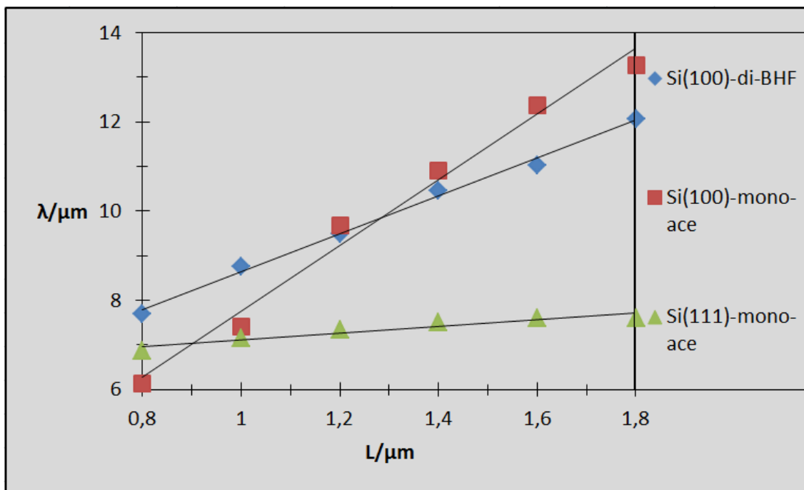
Obrázek 8.9: Srovnání rezonančních vlnových délek pro pole antén vyrobených metodou FIB pro dimery na Si(100) rezistivity 6 - 9 \Omega \cdot \text{cm} ošetřeného BHF s vrstvou titanu, monomery na křemíkovém substrátu Si(100) rezistivity 6 - 9 \Omega \cdot \text{cm} ošetřeného acetonem s vrstvou titanu a monomery na křemíkovém substrátu Si(111) rezistivity 10^{-3} \Omega \cdot \text{cm} s vrstvou titanu.
