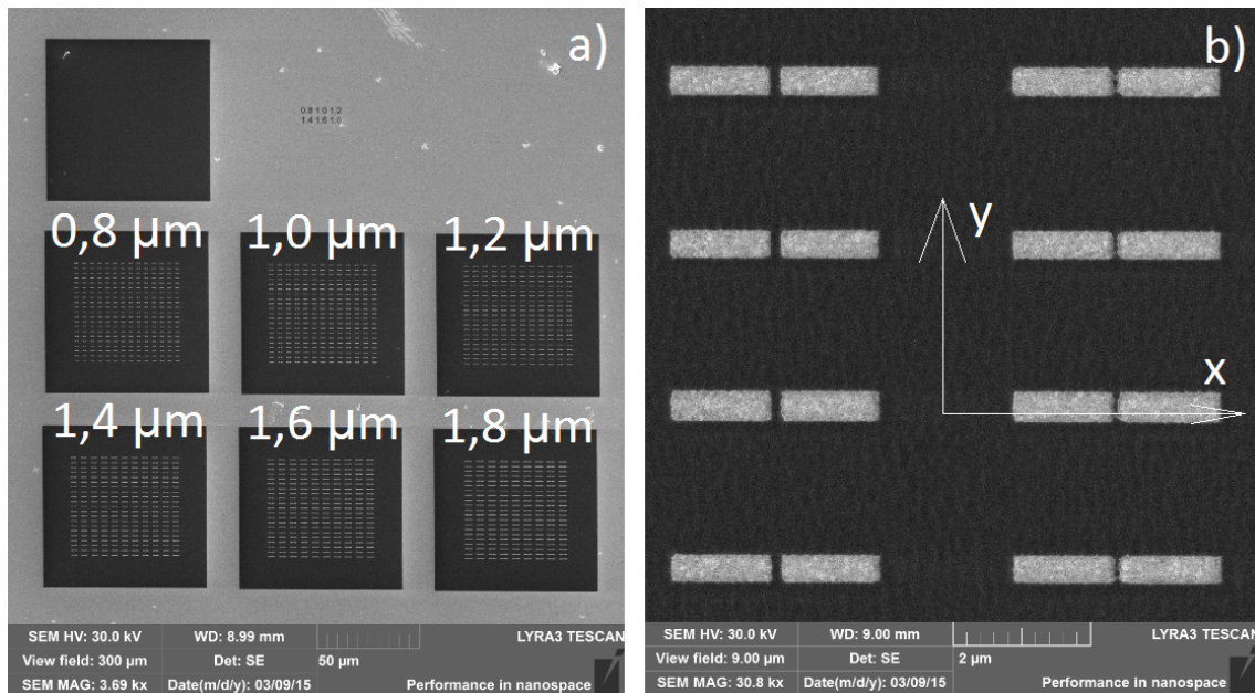
Obrázek 8.3: a) obrázek vzorku zlatých antén na křemíkovém substrátu Si(100) rezistivity 6 - 9 \Omega \cdot \text{cm} ošetřeného BHF s vrstvou titanu vyrobených metodou FIB pořízený pomocí rastrovacího elektronového mikroskopu. Vlevo nahoře je prázdné pole (čistý křemík) sloužící k měření pozadí, další pole jsou s anténami různých délek. b) detail antény délky 1,2 \mu\text{m} .
