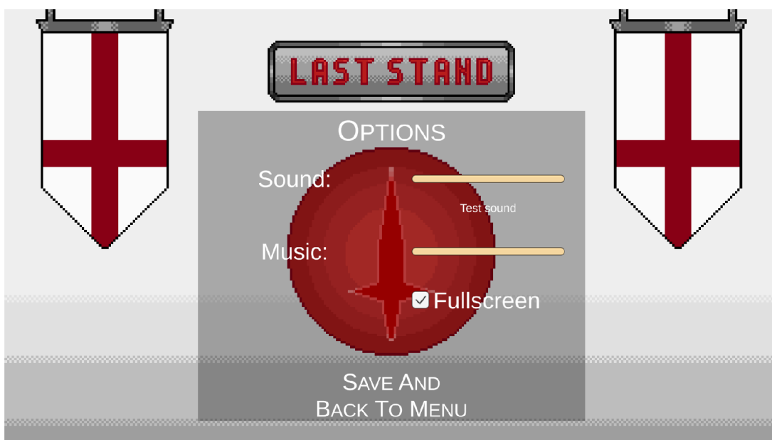
Obrázek 7: Nastavení
