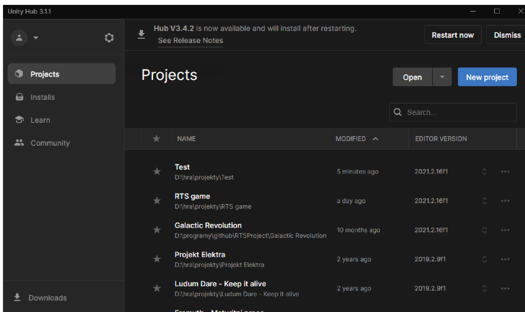
Obrázek 1: UnityHub
