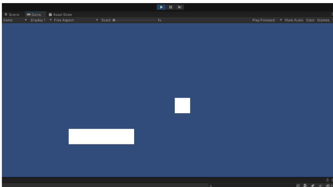
Obrázek 5: Spuštěná scéna
