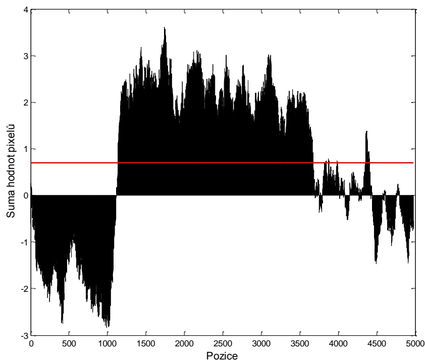
Obr. 17: Rozdíl sumovaných spekter zeleného a červeného spektrogramu DNA sekven- ce (chromozomu 21 člověka, hs_alt_CHM1_1.1_chr21:25000-30000 ), stanovená pra- hová hodnota je označena červenou barvou. Začátek CpG ostrůvek byl v tomto případě algoritmem CpGI stanoven na pozici 1134, konec na pozici 3676, tedy o délce 2542 bp.
