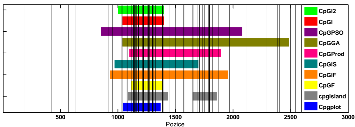
Obr. 26: Porovnání nalezených CpG ostrůvků lokalizovaných jednotlivými vyhledávači v DNA sekvenci genu somatostatin I ( seq_5.fasta ). Svislé čáry zobrazují výskyt CpG na konkrétní pozici v sekvenci.
