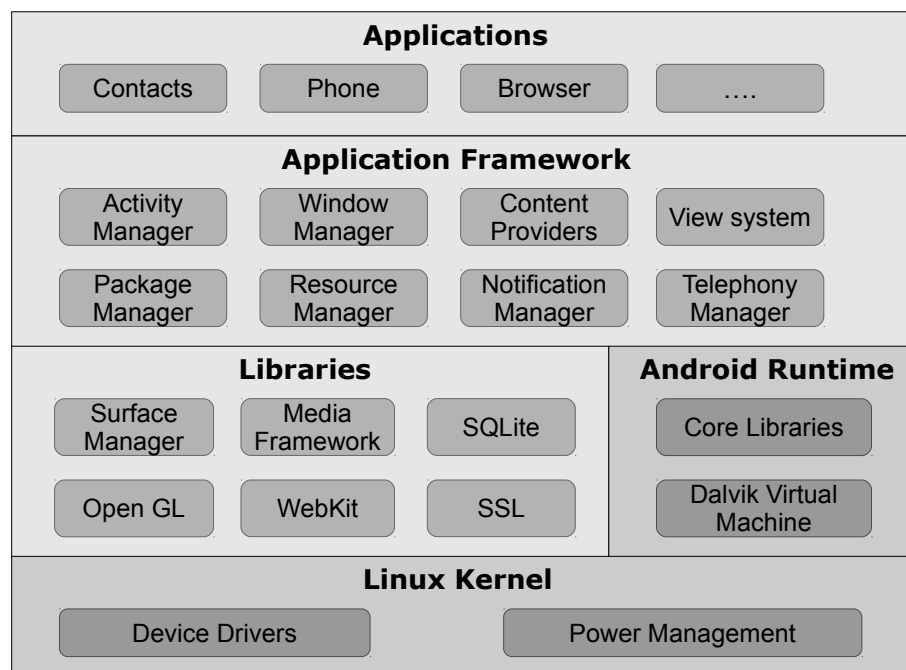
Obrázek 2.1: Achitektura systému Android.
