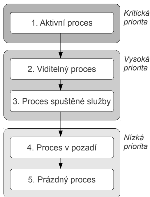
Obrázek 2.2: Stavy procesů.
