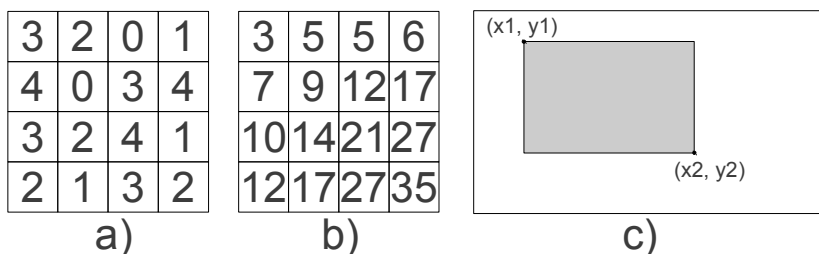
Obrázek 3.3: Integrální obraz. a) vstupní matice. b) vypočítaný integrální obraz. c) použití integrálního obrazu k výpočtu sumy šedé oblasti.
