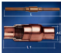
Obrázok 2. 9 - Parametre kompenzačnej vsuvky [33]
