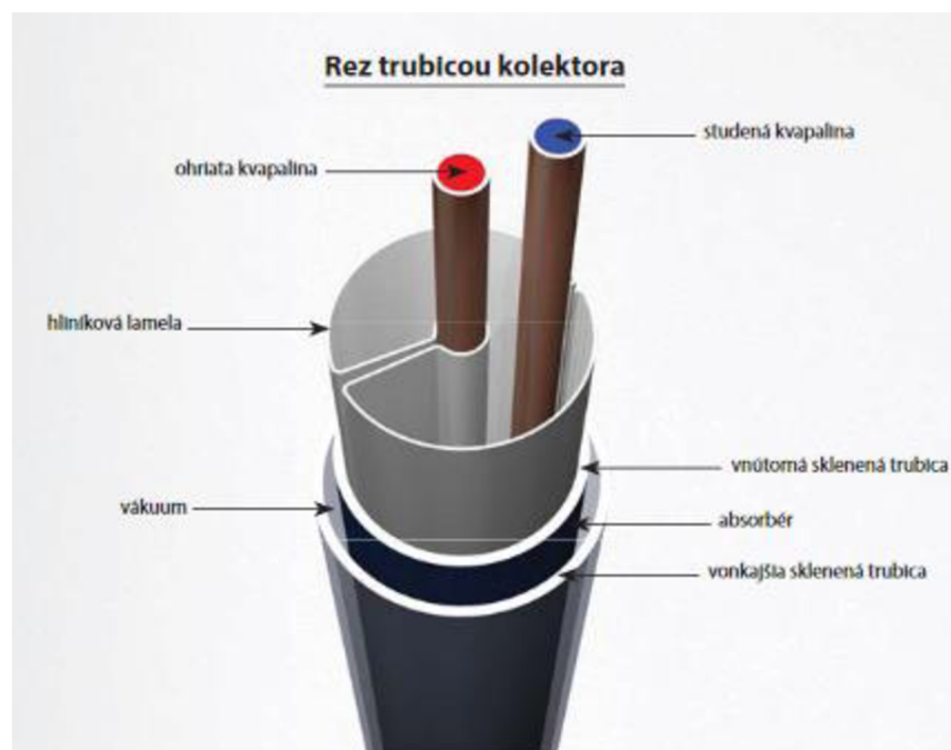
Obrázok 1. 12 – Rez priamo pretekaným trubicovým kolektorom [15]
