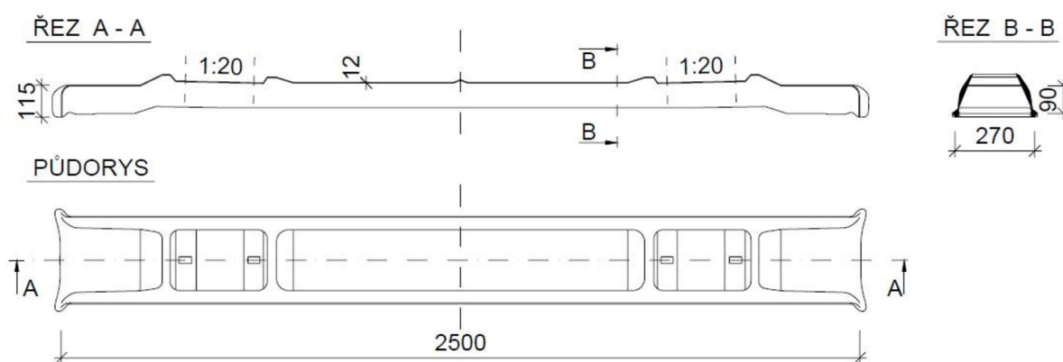
Obr. 3.2.3 Ocelový pražec T 3 [4]
