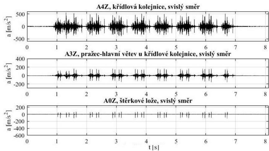
Obr. 6.2.6 Srovnání grafů zrychlení vibrací, výhybky č. 3 a 4 při průjezdu vlakových souprav RailJet
