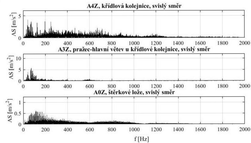
Obr. 6.3.3 Srovnání grafů zrychlení vibrací ve frekvenčním spektru, výhybky č. 3 a 4 při průjezdů vlakových souprav 380 a RegioJet
