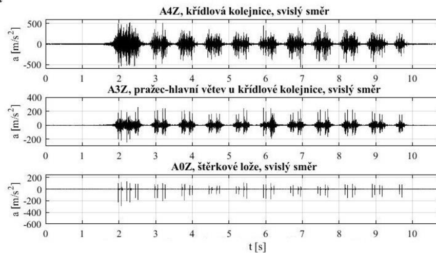
Obr. 6.2.5 Srovnání grafů zrychlení vibrací, výhybky č. 3 a 4 při průjezdů vlakových souprav 380 a RegioJet
