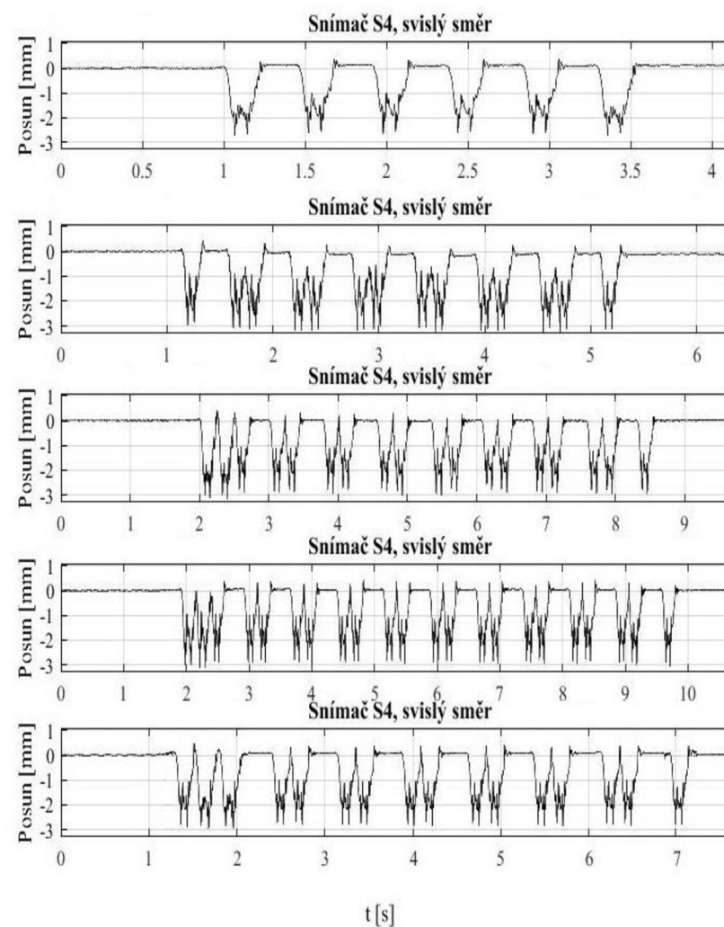
Obr. 6.1.4 Srovnání grafů průhybu pražce pod srdcovkou výhybky při průjezdu vlakových souprav, shora dolů v řádcích: LEO Express, Pendolino, lokomotiva řady 380, RegioJet, Railjet.
