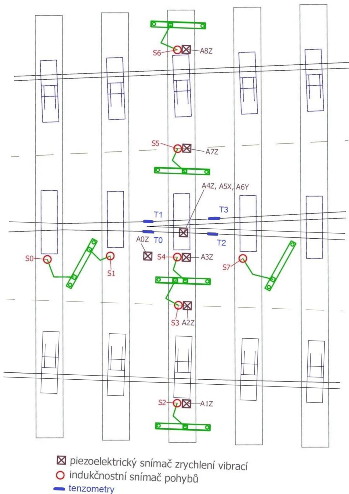
Obr. 4.4 Schéma rozmístění snímačů [7]
