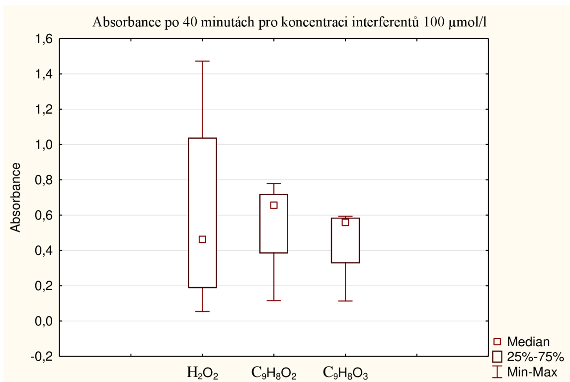
Obr. 34: Absorbance peroxidu vodíku a interferujících kyselin o koncentraci 100 \mu\text{mol/l} po 40 minutách pro metodu s KI při vlnové délce 390 nm
