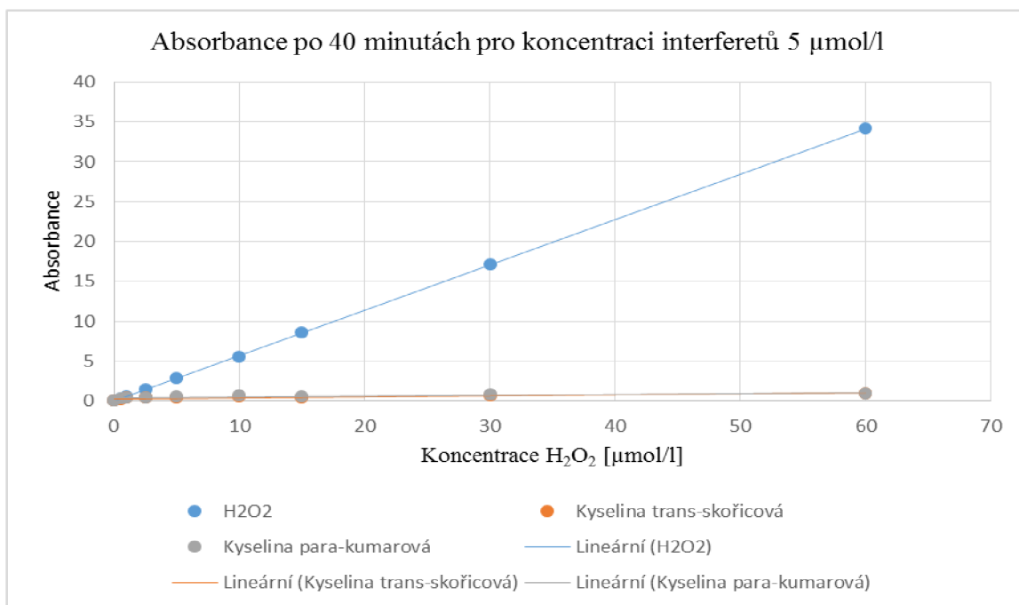
Obr. 26: Absorbance peroxidu vodíku a interferujících kyselin o koncentraci 5 \mu\text{mol/l} po 40 minutách pro metodu s KI při vlnové délce 390 nm
