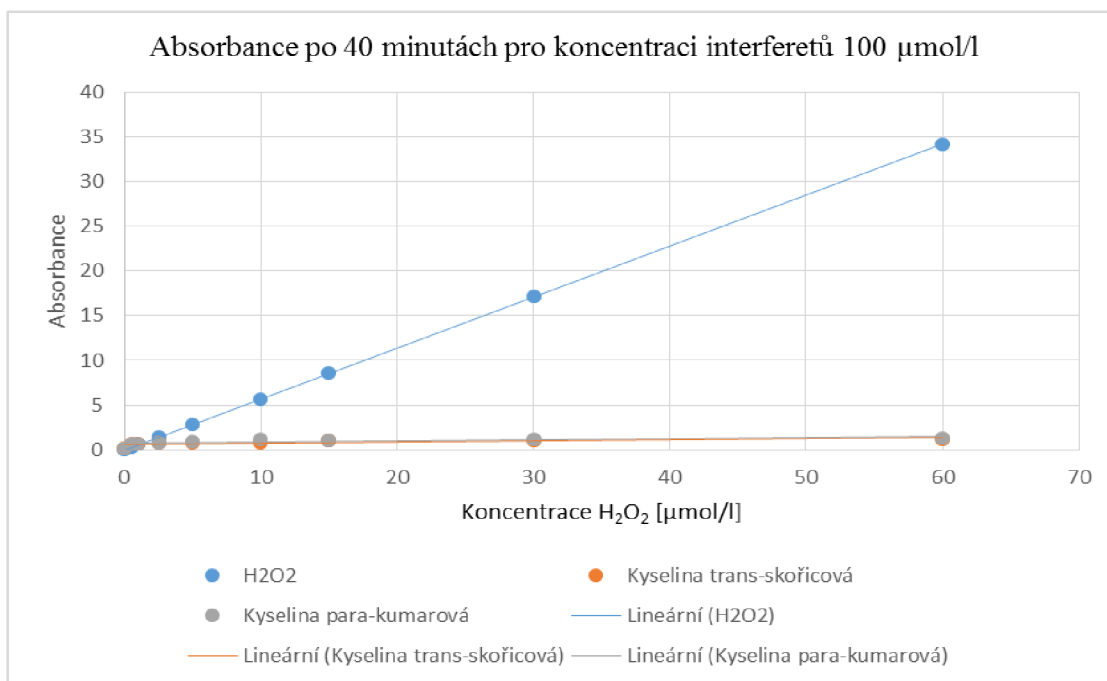
Obr. 34: Absorbance peroxidu vodíku a interferujících kyselin o koncentraci 100 \mu\text{mol/l} po 40 minutách pro metodu s KI při vlnové délce 390 nm
