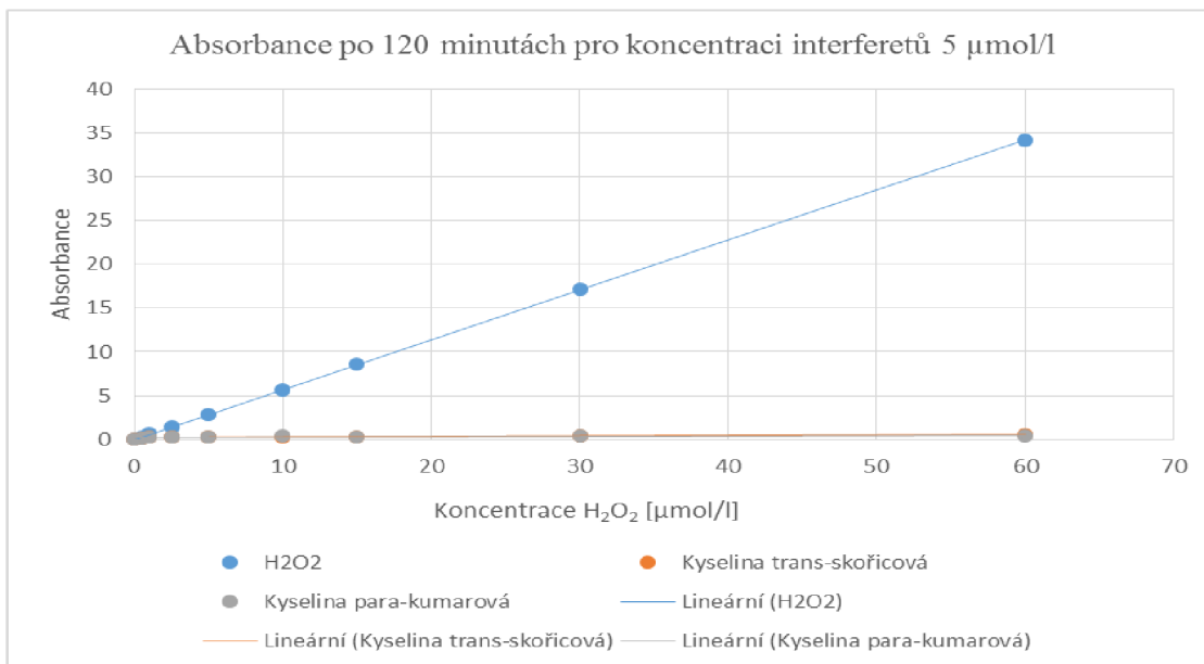
Obr. 24: Absorbance peroxidu vodíku a interferujících kyselin o koncentraci 5 μmol/l po 120 minutách pro metodu s KI při vlnové délce 410 nm
