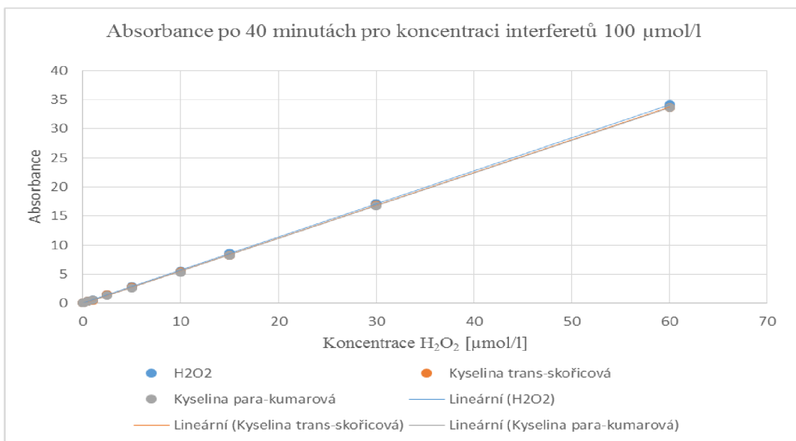
Obr. 16: Absorbance peroxidu vodíku a interferujících kyselin o koncentraci 100 μmol/l po 40 minutách pro metodu s TiCl 4 při vlnové délce 390 nm
