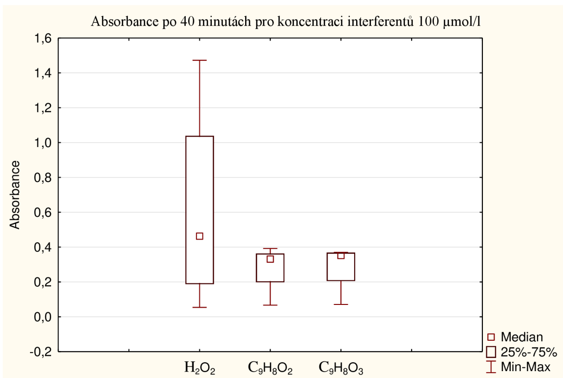
Obr. 30: Absorbance peroxidu vodíku a interferujících kyselin o koncentraci 100 \mu\text{mol/l} po 40 minutách pro metodu s KI při vlnové délce 410 nm
