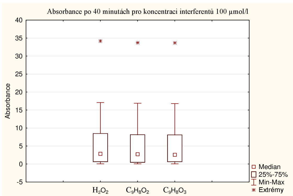
Obr. 17: Rozložení hodnot absorbance po 40 minutách pro oba interferenty o koncentraci 100 μmol/l pro TiCl 4 (390 nm)
