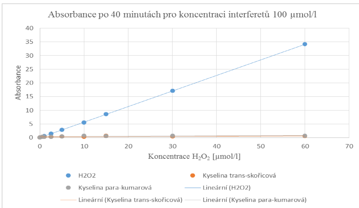
Obr. 30: Absorbance peroxidu vodíku a interferujících kyselin o koncentraci 100 \mu\text{mol/l} po 40 minutách pro metodu s KI při vlnové délce 410 nm
