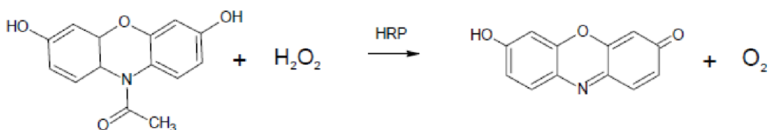
Rovnice 7: Reakce Amplex Red s peroxidem vodíku, převzato z: [III]
