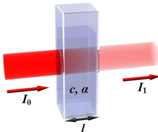
Obr. 1: Absorbance, převzato z: [1]
