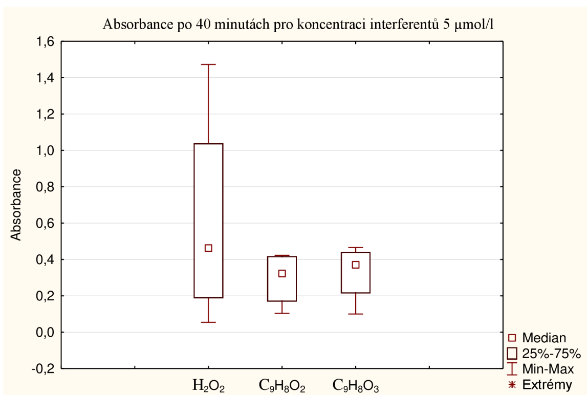
Obr. 26: Absorbance peroxidu vodíku a interferujících kyselin o koncentraci 5 \mu\text{mol/l} po 40 minutách pro metodu s KI při vlnové délce 390 nm
