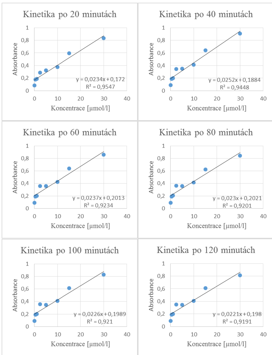
Obr. 21: Kalibrační křivky standardu ( \text{H}_2\text{O}_2 ) pro KI metodu (390 nm)
