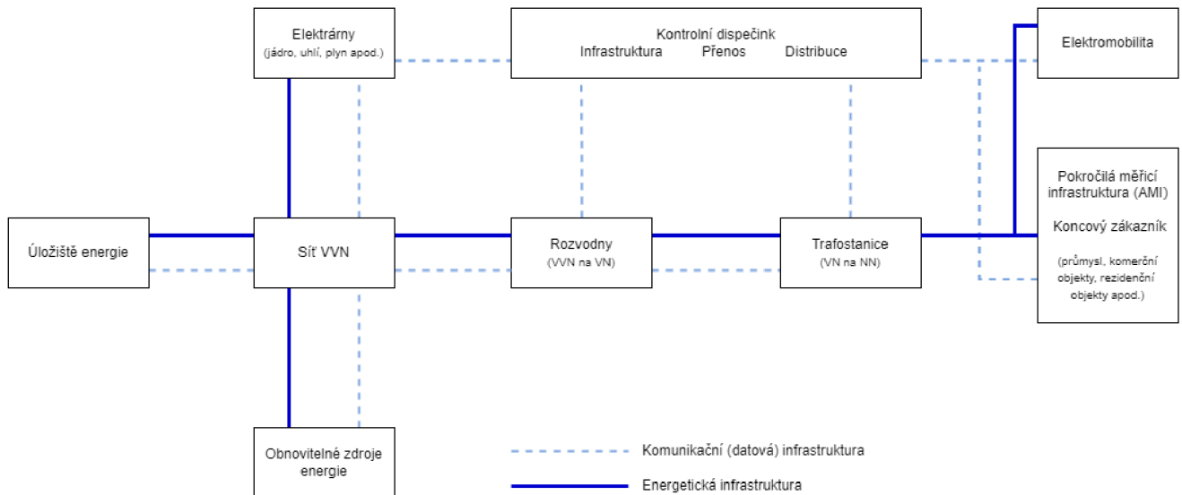
Obrázek 11 - Blokové schéma technologie Smart Grid, zdroj: autor
