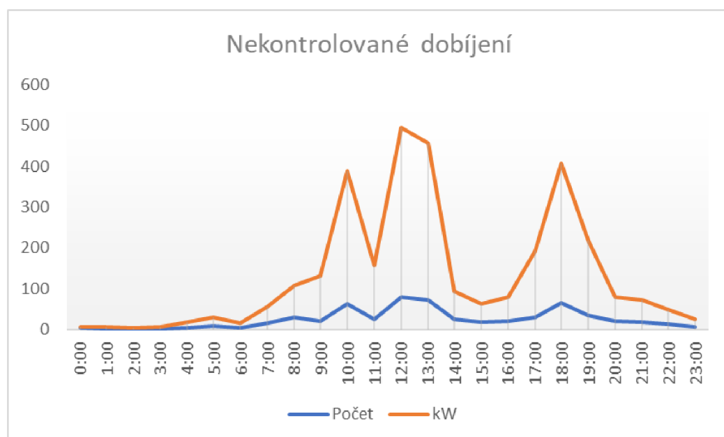
Obrázek 1 - Graf špiček nekontrovaného dobíjení, zdroj: autor
