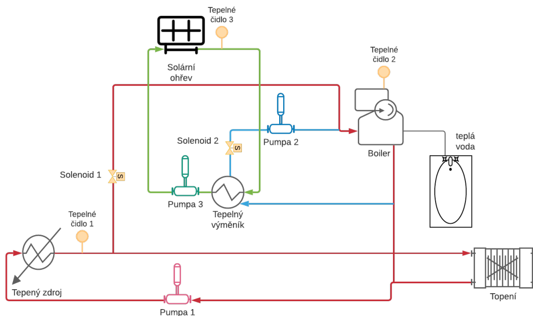
Obrázek 3.1: Schéma aktuálního systému. Systém obsahuje bojler a dva externí zdroje. První zdroj je teplovodní okruh vytápění domu. Ten je ohříván kamny na dřevo. Druhým zdrojem je teplovodní okruh solárních panelů.
