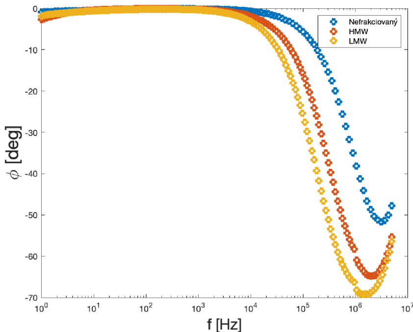
Obrázek 5.12: Bäckhammer Bodeho graf fázového posunu
