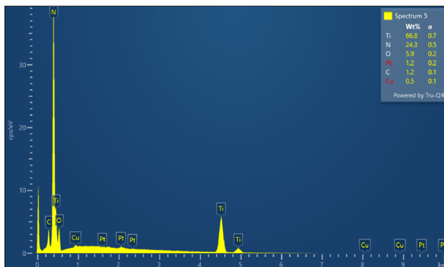
Obrázek 5.27: Spektrum TiON klastru na vlákně vrstvě
