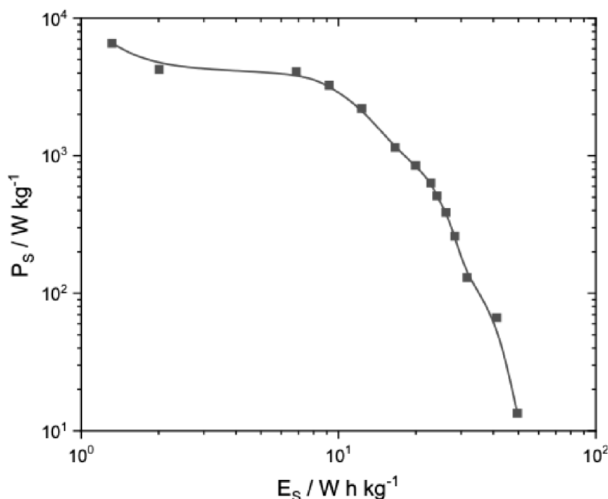
Obrázek 5.21: Specifický výkon vztažený na hmotnost
