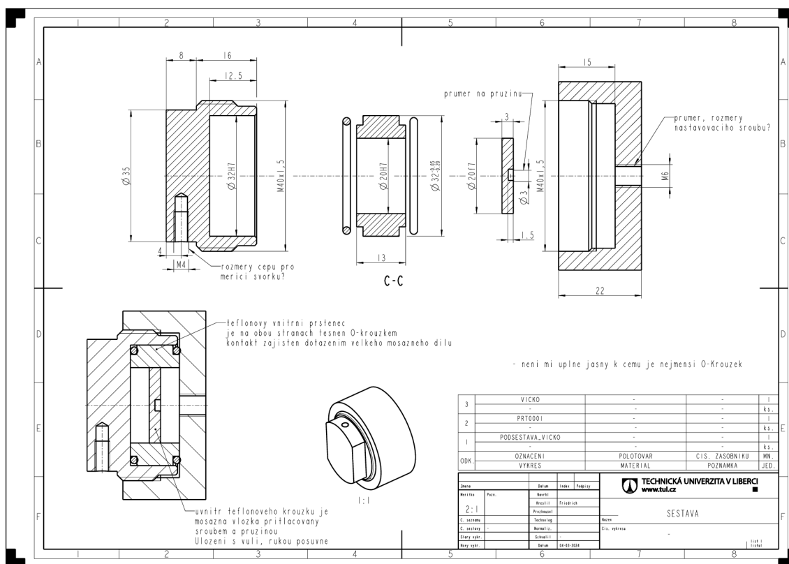
Obrázek 5.29: Držák pro dvouelektrokové měření kapacitorů
