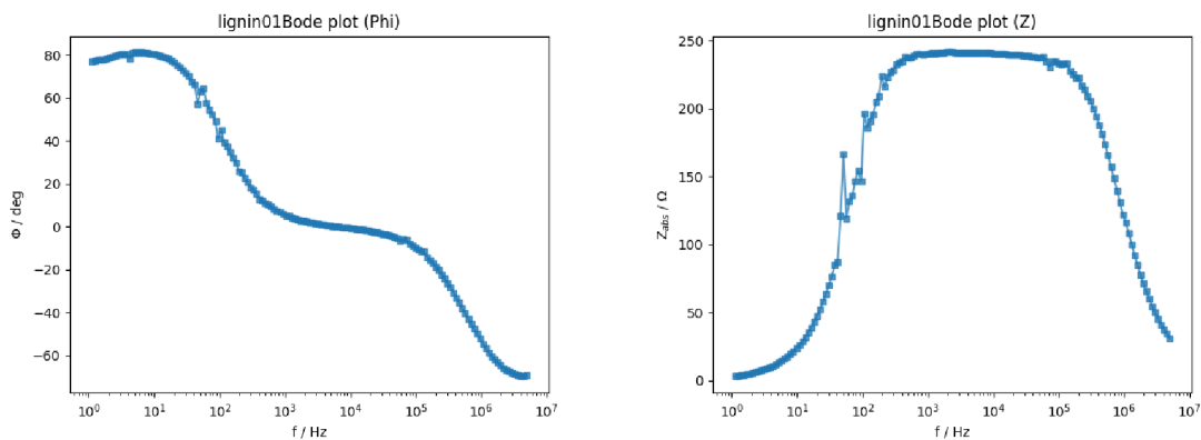
(a) Bodeho graf úhlu
