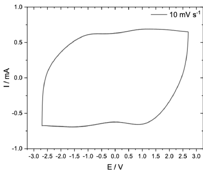
Obrázek 5.19: Závislost proudu na napětí
