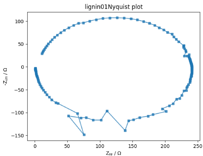
(c) Nyquistův graf
