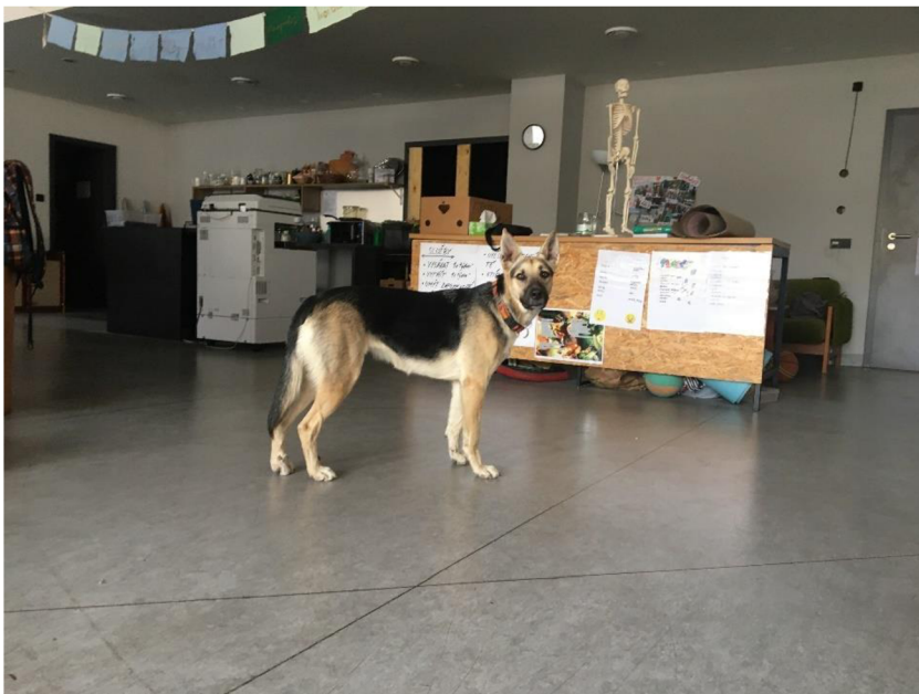
Obrázek 35 Rozložení třídy
