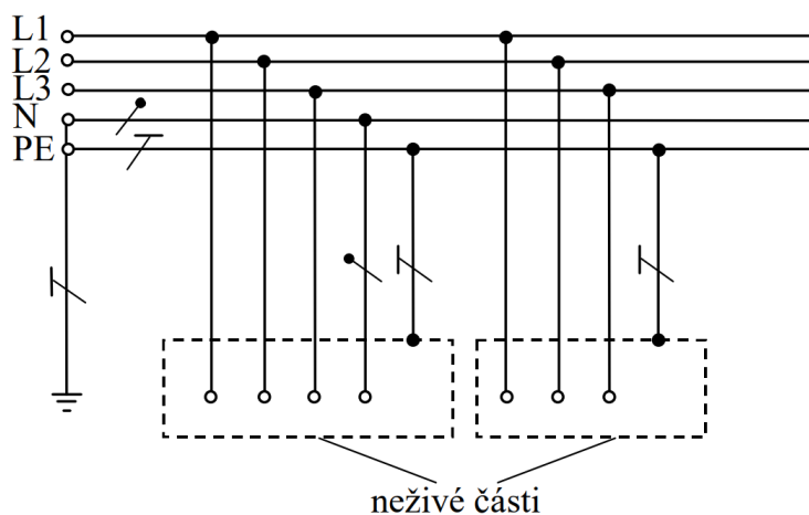
Obr. 2.2: Síť TN-S [7]
