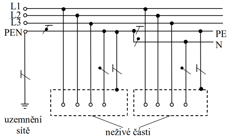
Obr. 2.3: Síť TN–C–S [7]
