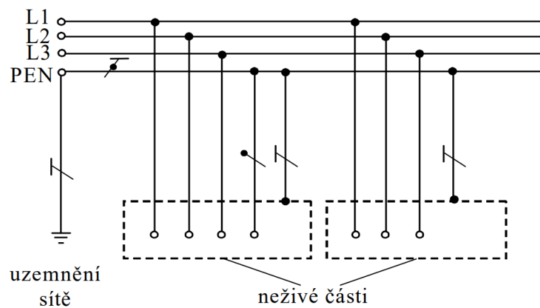
Obr. 2.1: Síť TN-C [7]
