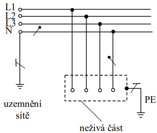
Obr. 2.5: Síť TT [7]
