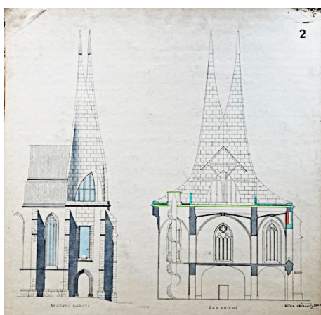
Obr. XXXIV. Řez průčelím kostela, 1965
