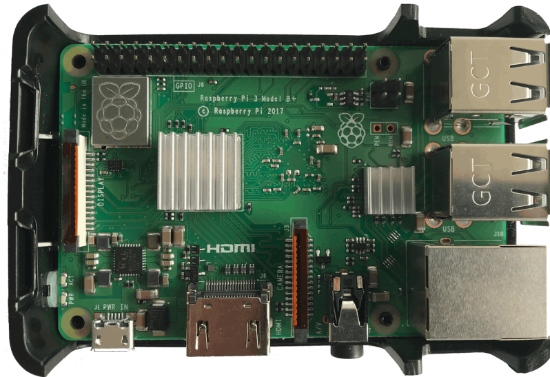
Obrázek 2.1: Raspberry Pi 3 Model B+ s přidaným pasivním chlazením umístěný v oficiální Raspberry Pi krabičce.
