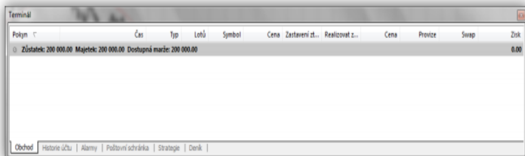
Obrázek 25: Okno terminál
