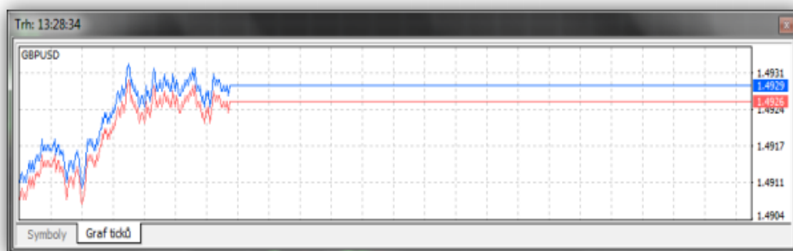
Obrázek 18: Graf ticků
