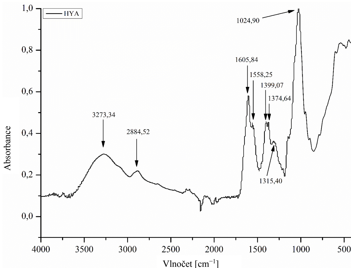
Obrázek 22 FTIR spektrum hyaluronanu (HYA)
