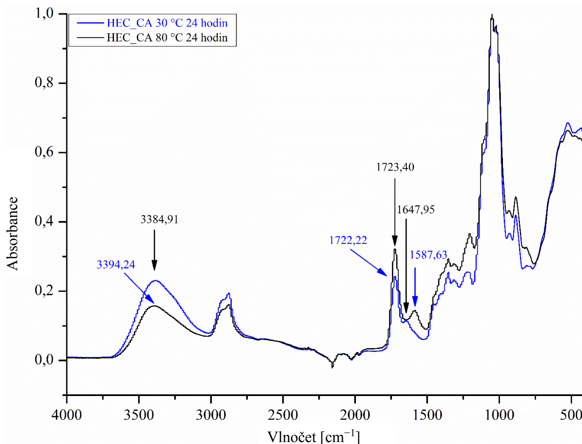
Obrázek 30 FTIR spektrum filmu 2% roztoku (w/w ultračisté deionizované vody) HEC s obsahem 20 % (w/w HEC) CA; po vysušení (30 °C) a po zesítní (80 °C)
