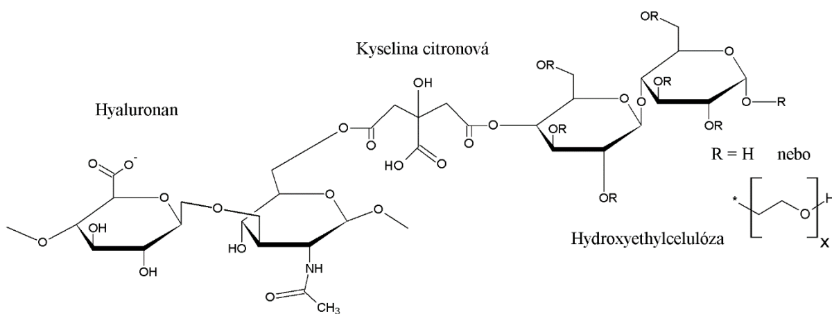
Obrázek 25 Znázornění možného zesíťení daných polymerů kyselinou citronovou
