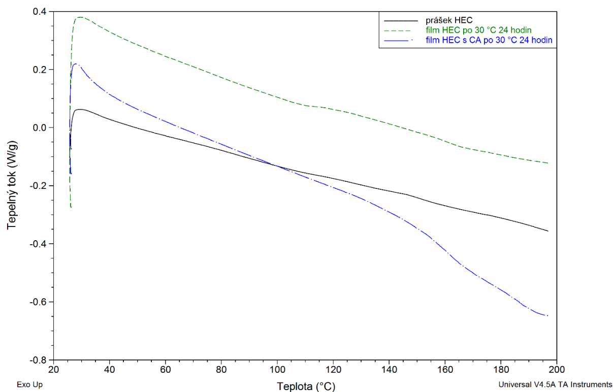
Obrázek 44 DSC záznam prášku hydroxyethylcelulózy (HEC), filmu HEC po 30 °C 24 hodin a filmu HEC a kyseliny citronové (CA) po 30 °C 24 hodin; 2. části cyklu měření
