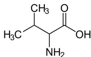
Obrázek 8: L-valin ( www.sigmaaldrich.com )
