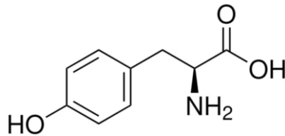
Obrázek 16: L-tyrosin ( www.sigmaaldrich.com )
