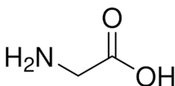
Obrázek 24: Glycin ( www.sigmaaldrich.com )
