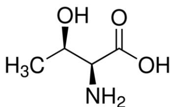
Obrázek 12: L-threonin ( www.sigmaaldrich.com )
