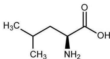
Obrázek 7: L-leucin ( www.sigmaaldrich.com )
