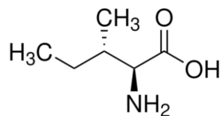
Obrázek 6: L-isoleucin ( www.sigmaaldrich.com )
