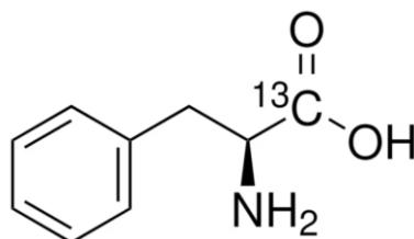
Obrázek 11: L-fenylalanin ( www.sigmaaldrich.com )
