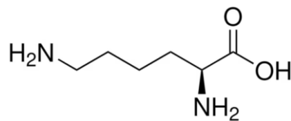
Obrázek 9: L-lysine ( www.sigmaaldrich.com )
