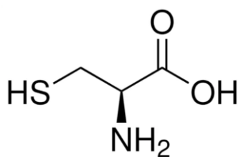
Obrázek 15: L-cystein ( www.sigmaaldrich.com )
