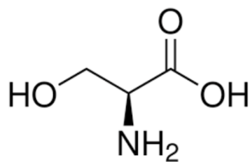
Obrázek 25: L-serin ( www.sigmaaldrich.com )
