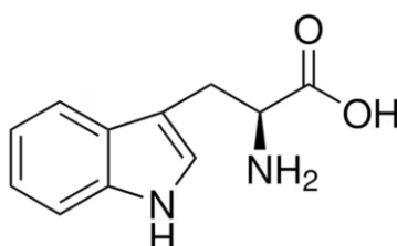
Obrázek 13: L-tryptofan ( www.sigmaaldrich.com )
