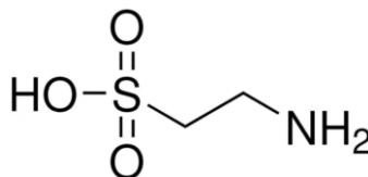
Obrázek 17: L-taurin ( www.sigmaaldrich.com )
