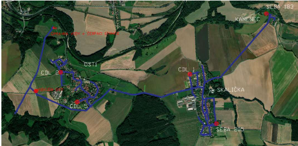
Obrázek 18. Mapa osazení tlakových čidel
