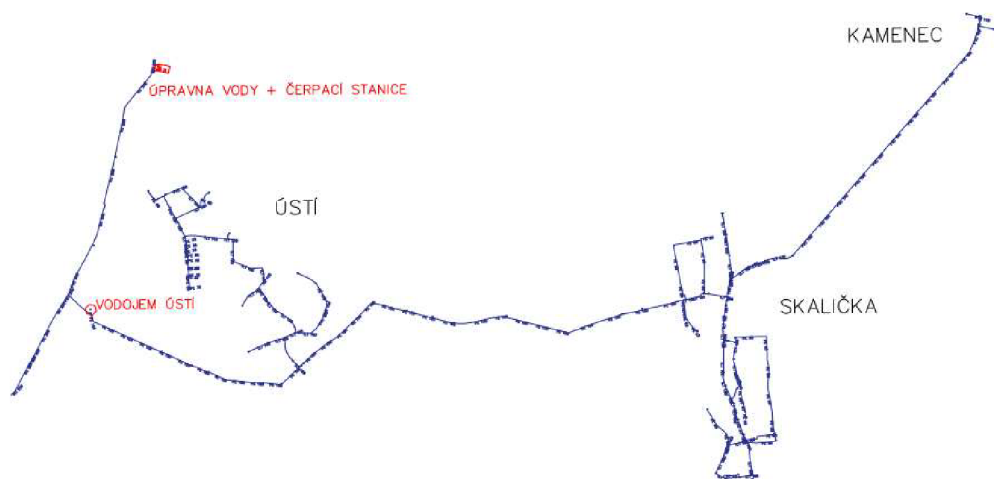
Obrázek 17. Schéma rozvodné sítě vodovodu v obcích
