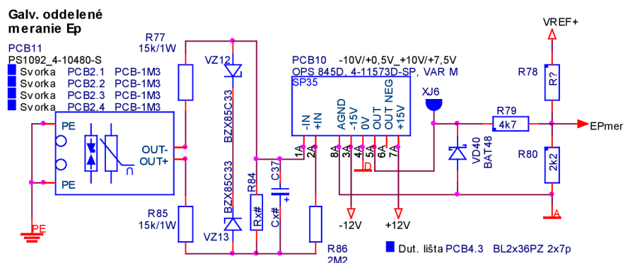
Obrázok 26:Galv. oddelené meranie potenciálu
