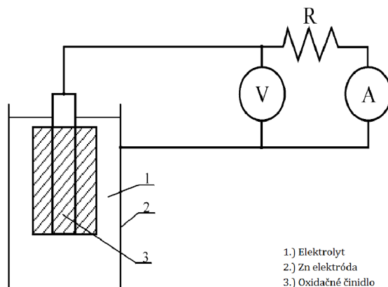
Obrázok 5: Mechanizmus elektrochemickej korózie
