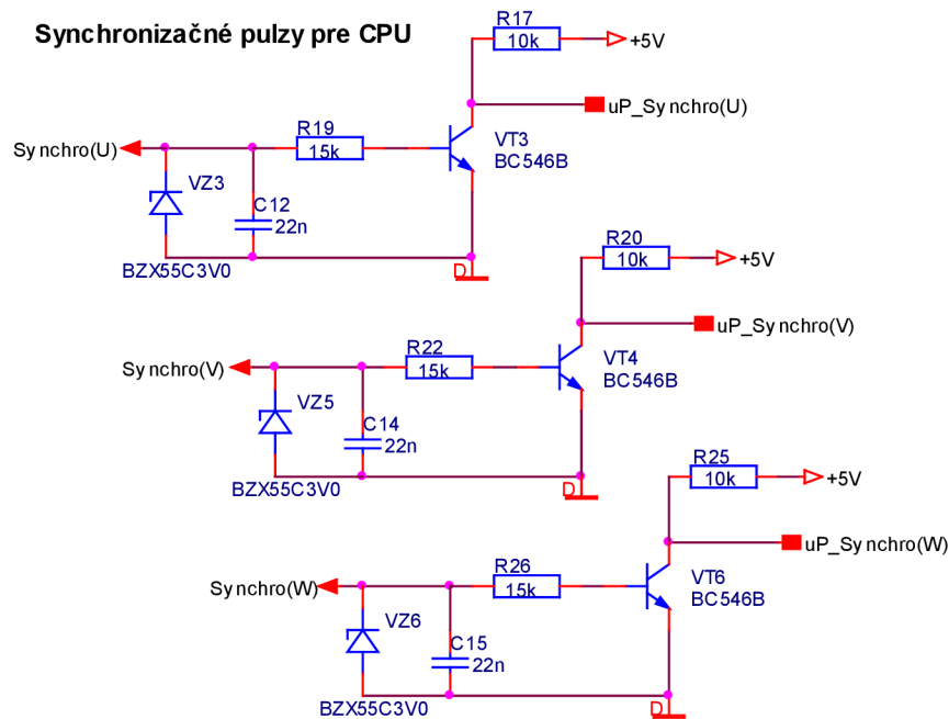
Obrázok 29. Synchronizačné pulzy
