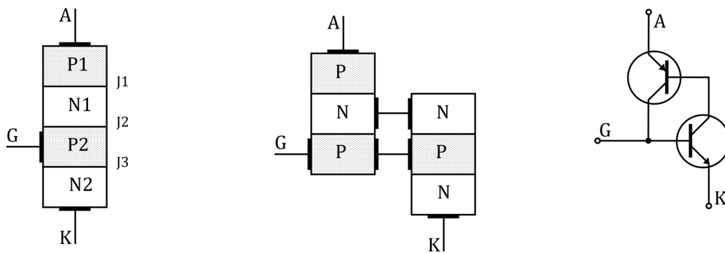
Obrázok 12: Základná štruktúra PNP. Myšlienkové rozdelenie na dve štruktúry. Obvodový model tyristoru
