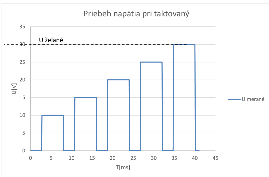
Graf 4: Dokonalý priebeh taktovanie
