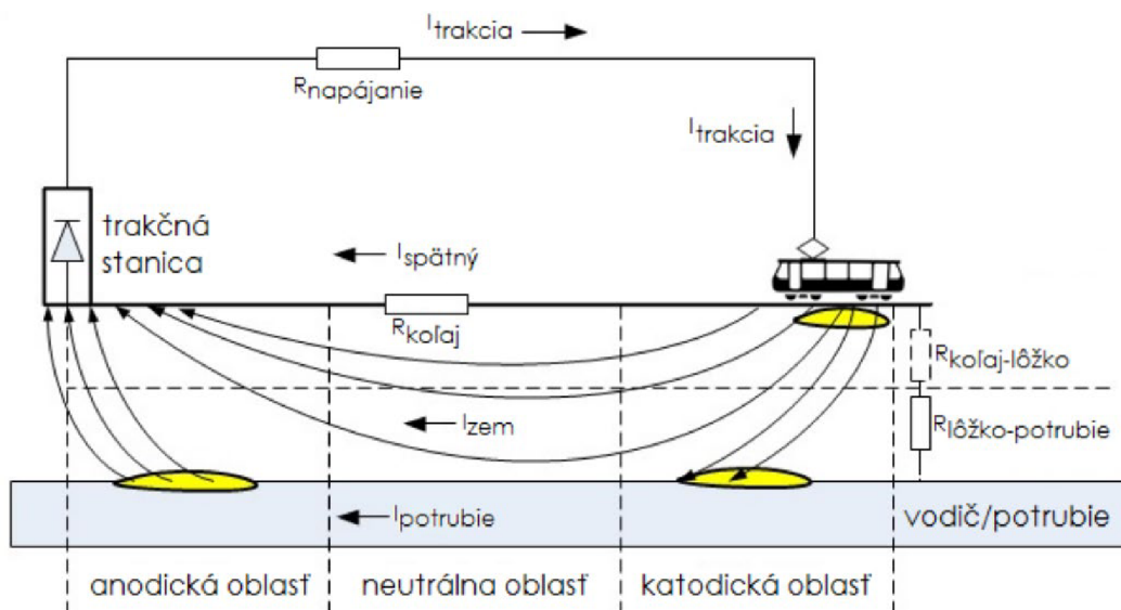
Obrázok 9: Oblasti pôsobenia blúdivých prúdov[10]
