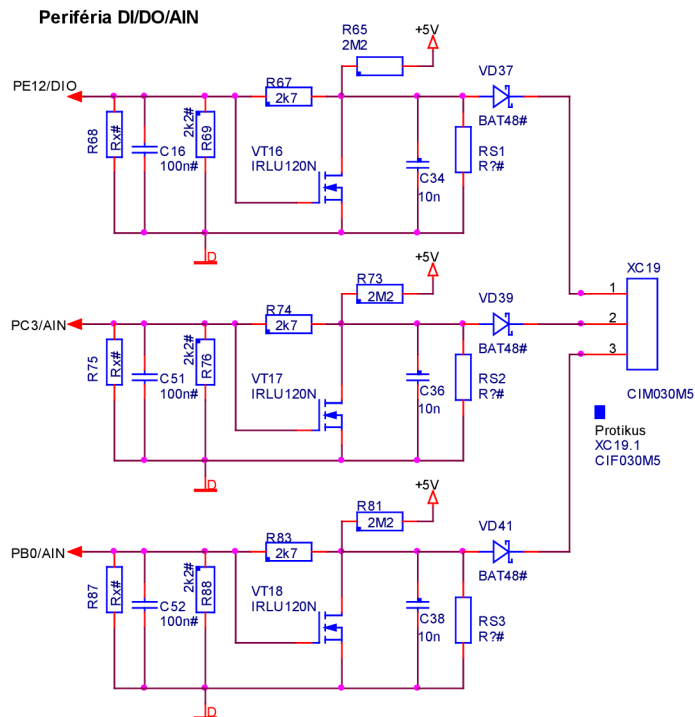
Obrázok 20: Zapojenie DO/DI/IA periférií
