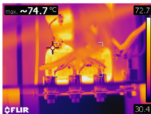
Obrázok 50: Termo kamera a.) vstupné poistky b.)Tyristory
