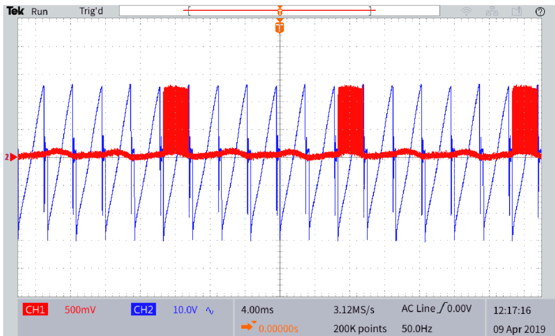
Graf 11: Zapaľovacie pulzy a rekuperácia (CH1 – Zapaľovacie pulzy, CH2 - Napätie pred výstupným filtrom )
