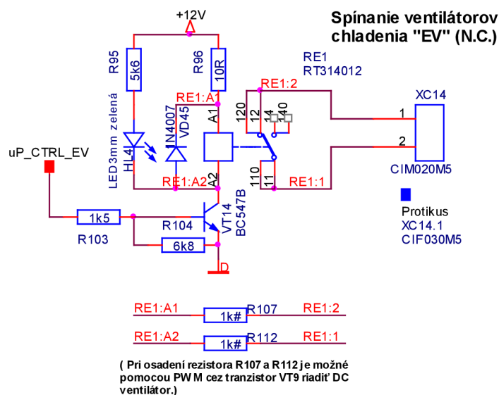
Obrázok 21:Ovládanie ventilátoru
