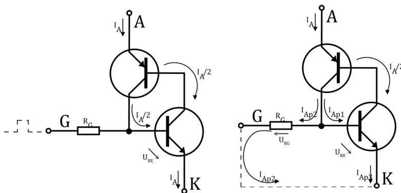
Obrázok 13: Vypnutie tyristora
