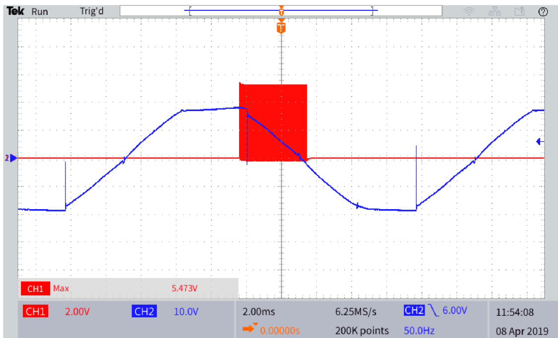
Graf 5: Synchronizácia tyristoru
