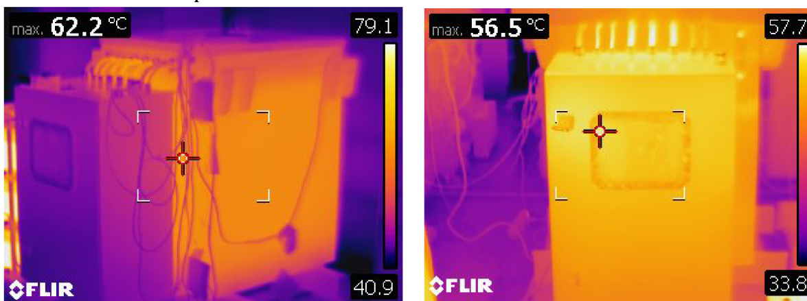
Obrázok 51: Termo kamera celé zariadenie
