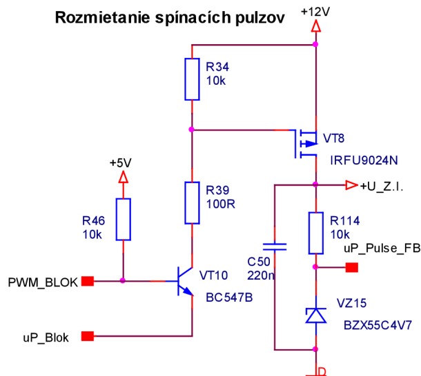
Obrázok 31: Blokovanie a rozmiestanie pulzov
