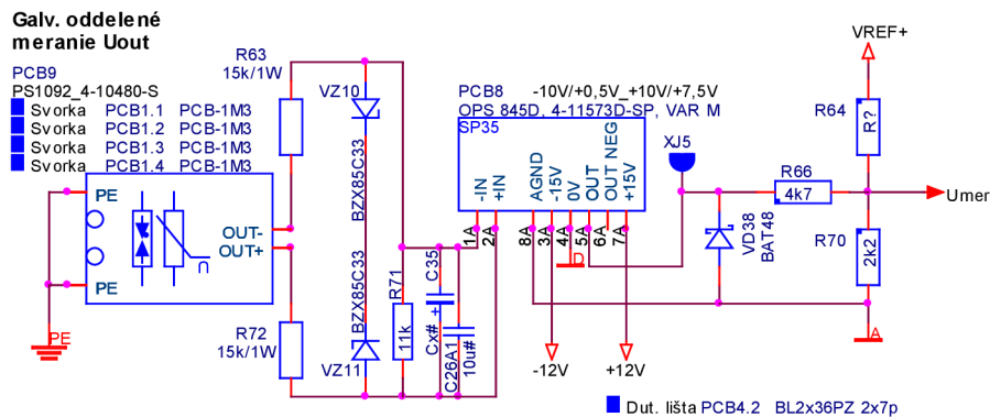
Obrázok 25:Galv. oddelené meranie napätia
