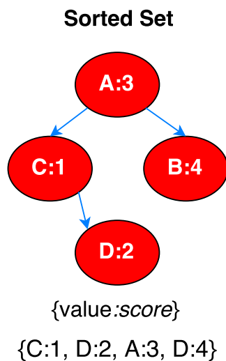
Obr. 2.10: Ukážka uloženia dátového typu sorted set databázy Redis
