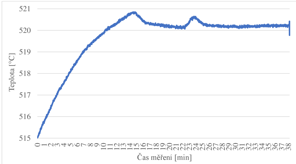
Obr. 32 Část průběhu teploty rozpouštěcího žihání
