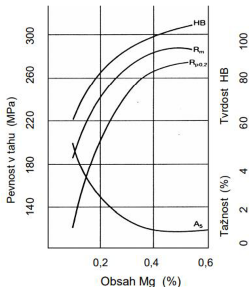
Obr. 23 Vliv Mg na mechanické vlastnosti po vytvrzení [2]
