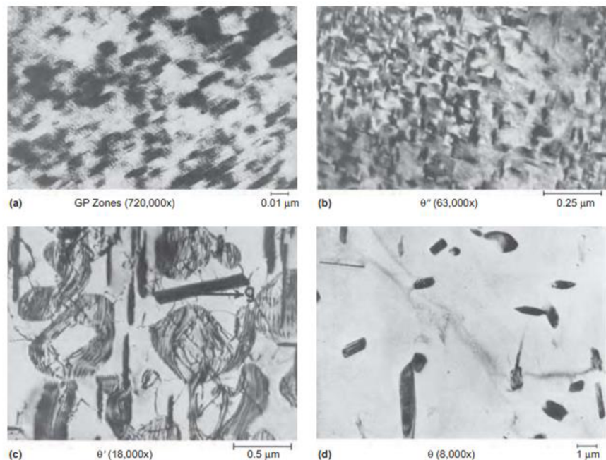
a) Guinier-Prestonovy zóny, b, c) semikoherentní precipitáty, d) nekoherentní precipitáty
