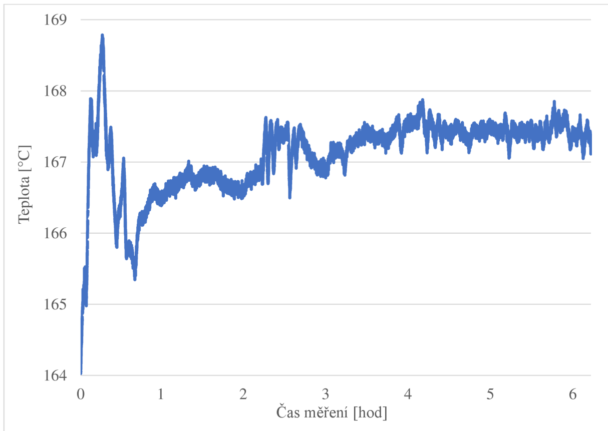
Obr. 35 Průběh teploty vytvrzování sady vzorků A
