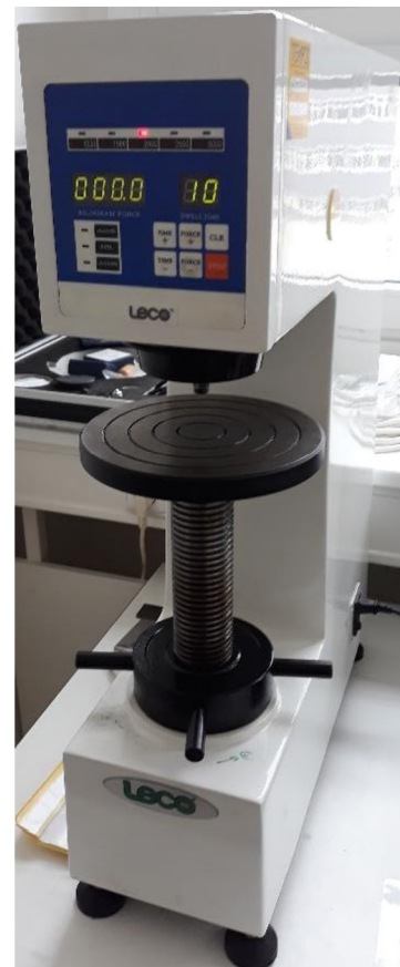
Obr. 40 Tvrdoměr
