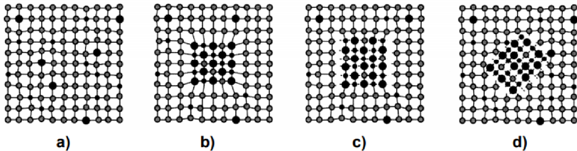
a) tuhý roztok, b) koherentní precipitát, c) semikoherentní precipitát, d) nekoherentní precipitát
