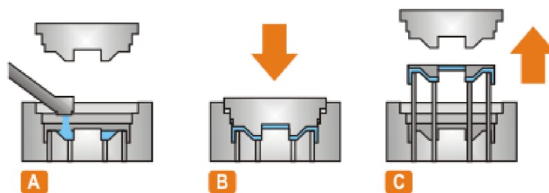
Obr. 15 Průběh přímého squeeze castingu [23]
