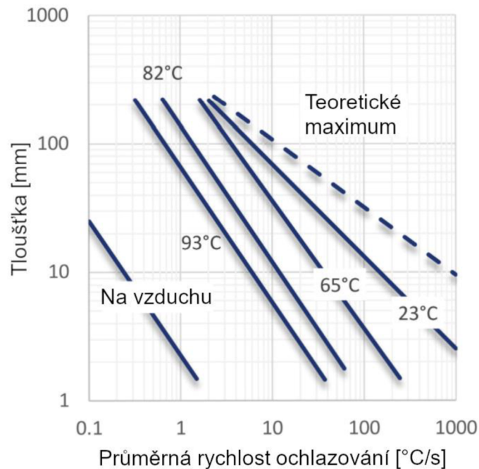
Obr. 19 Vliv teploty vodní lázně na rychlost ochlazování [27]
