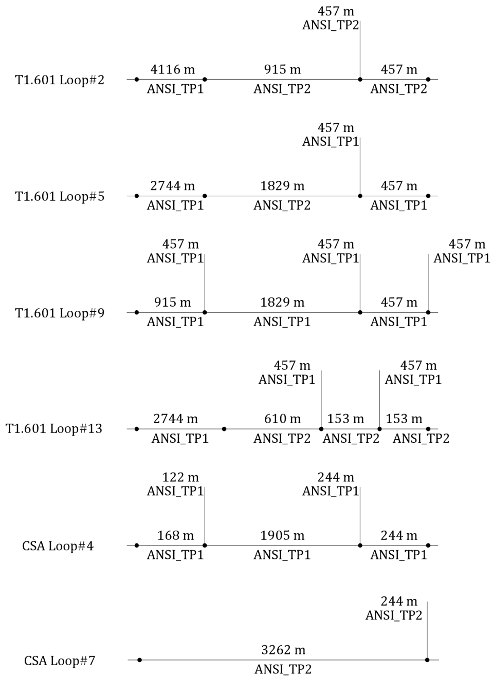
Obr. 4.9: Štruktúry testovacích ANSI smyčiek
