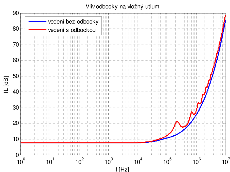
Obr. 4.4: Vliv odbočky na vložný útlum vedení; úsek vedení – kroucený pár ANSI_TP1, d = 0,4 \text{ mm} , l = 1 \text{ km} ; odbočka – kroucený pár ANSI_TP1, d = 0,4 \text{ mm} , l = 0,2 \text{ km}
