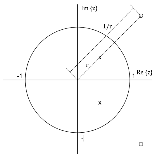
Obr. 5.2: Návrh fázovacího članku
