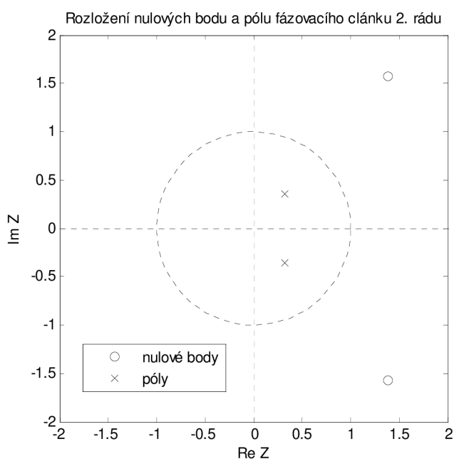
Obr. 5.3: Rozložení nulových bodů a pólů fázovacího članku 2. řádu
