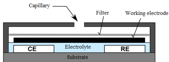
Fig. 18 Quasi-plannar structure
