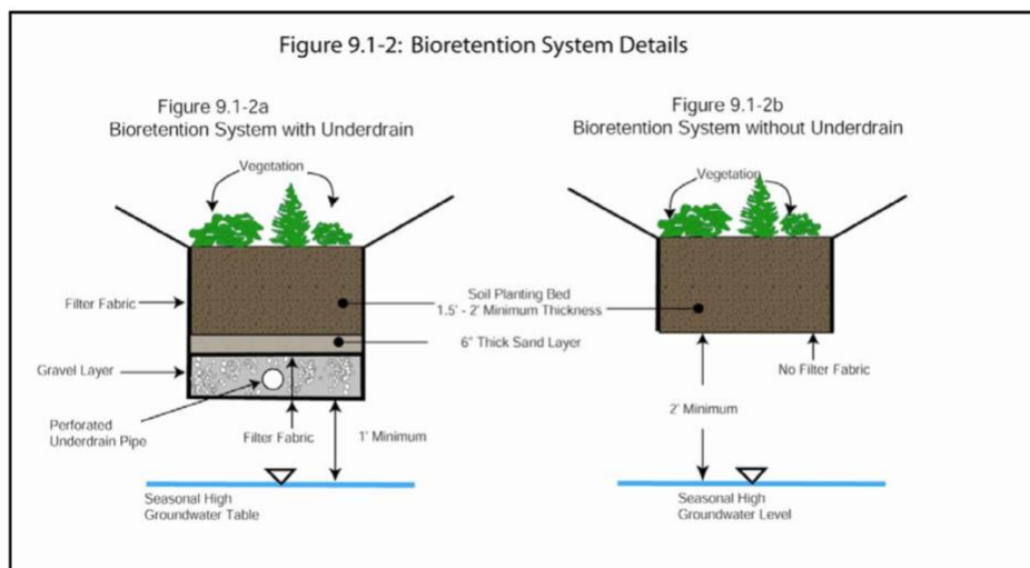
Obrázek 3: Bioretenční systém s odvodním kanálem a bez něj (State of New Jersey © 2009)
