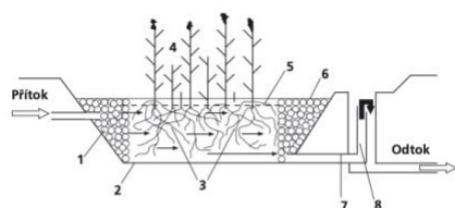
Obr. 2. Typické uspořádání kořenové čistírny. 1 – distribuční zóna (kamenivo, 50–200 mm), 2 – nepropustná bariéra (PE nebo PVC), 3 – filtrační materiál (kačírek, šterk, drcené kamenivo), 4 – vegetace, 5 – výška vodní hladiny v kořenové loži nastavitelná v odtokové šachtě, 6 – odtoková zóna (shodná s distribuční zónou), 7 – sběrná drenáž, 8 – regulace výšky hladiny
