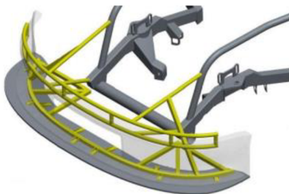
Obr. 23 Názorná poloha a umiestnenie splitteru na automobile [12]
