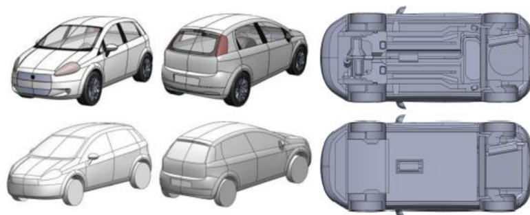
Obr. 19 Referenčný model Fiat Grande Punto [89]
