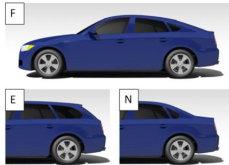
Obr. 8 DrivAer varianty Fastback (hore), Estateback (dole vľavo) a Notchback (dole vpravo) [12]
