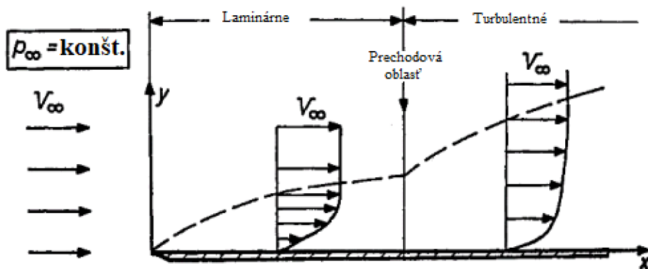
Obr. 2 postupný prechod z oblasti laminárneho prúdenia do oblasti turbulентného prúdenia [2]
