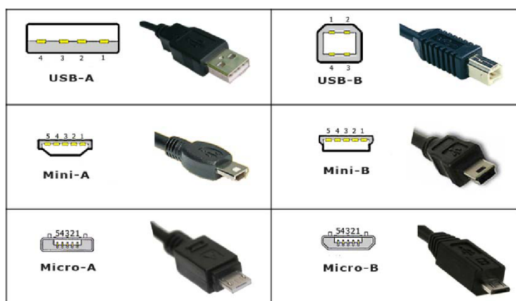
Obr. 2.3: Standardizované konektory USB kabelů
