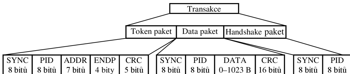
Obr. 2.4: Struktura paketů transakce na USB sběrnici
