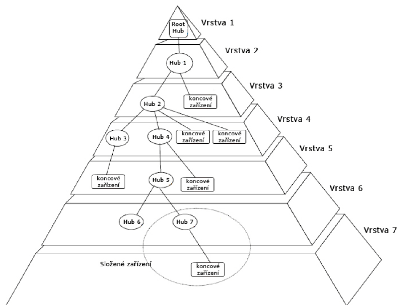
Obr. 2.2: Topologie USB sběrnice (převzato a upraveno z [7])
