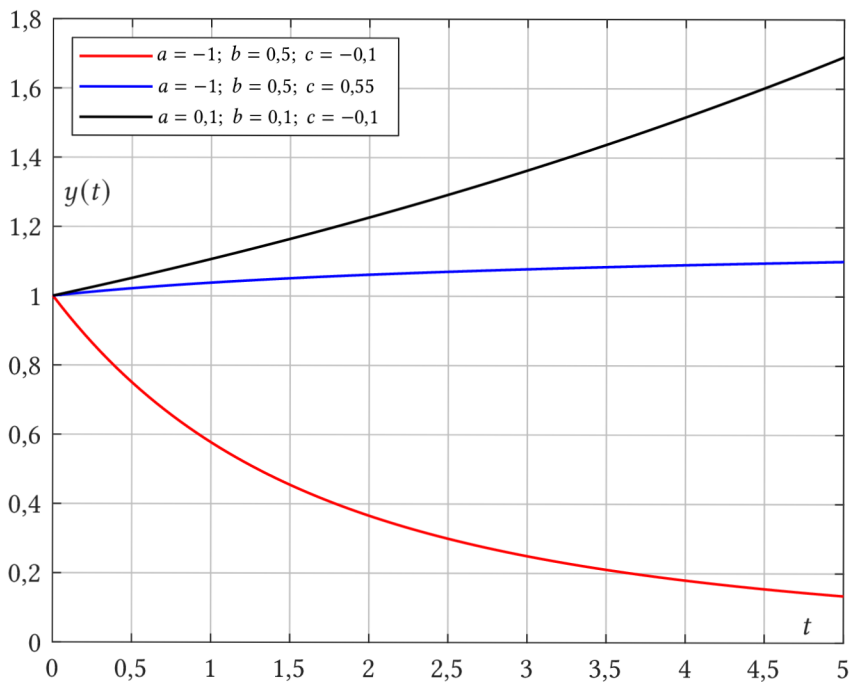
Obr. 10: Průběhy řešení pro q = 0,5; m = 2; l = 1; \phi = 1; t_0 = 0
