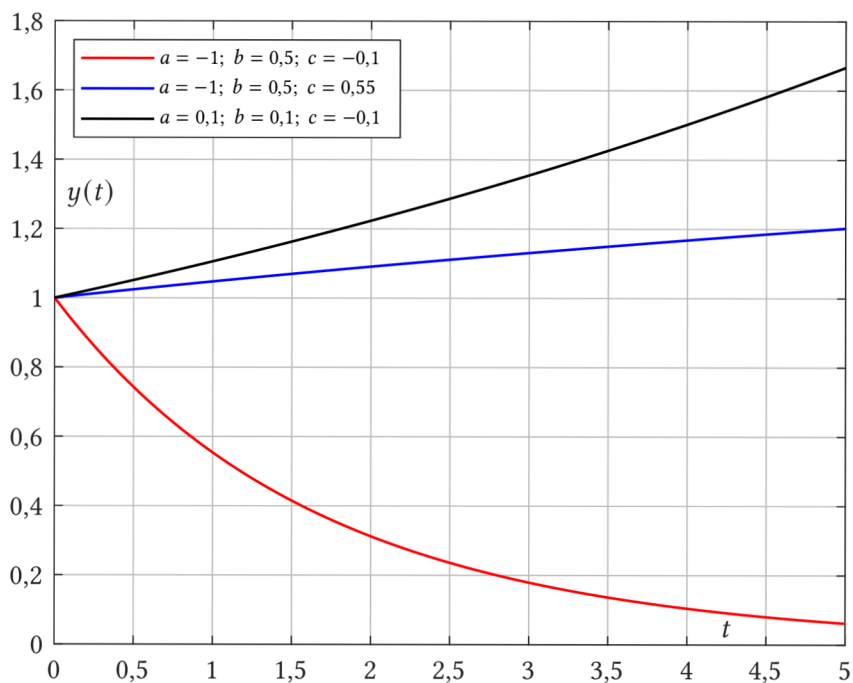
Obr. 9: Průběhy řešení pro q = 0,9; m = 2; l = 1; \phi = 1; t_0 = 0
