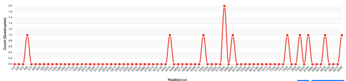
Obrázek 14: Závislost počtu G4 na pozici
