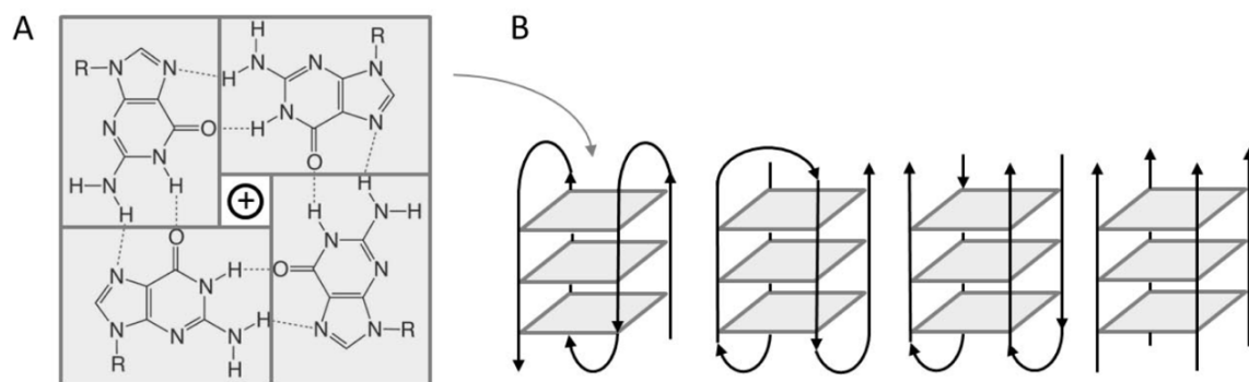
Obrázek 6: Obrázek 5: Guaninová tetráda a příklady G-kvadruplexu tvořeného jedním nebo více vláknů nukleových kyselin. Obrázek A – guaninová tetráda vytvořená na základě Hoogsteenova párování bází, Obrázek B – vrstvení guaninových tetrád a příklady G-kvadruplexů z jednoho, dvou a čtyř vláken nukleové kyseliny [89]
