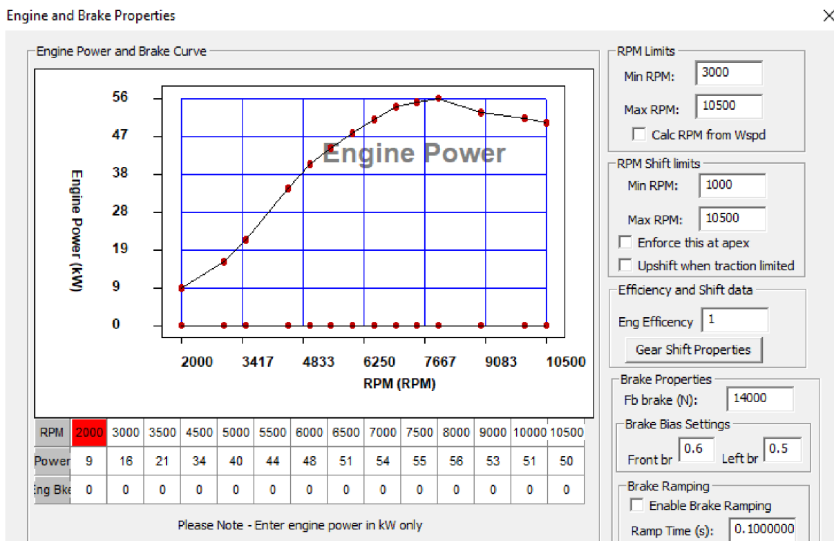
Obr. 47 Definícia spaľovacieho motora s E-Compressorom
