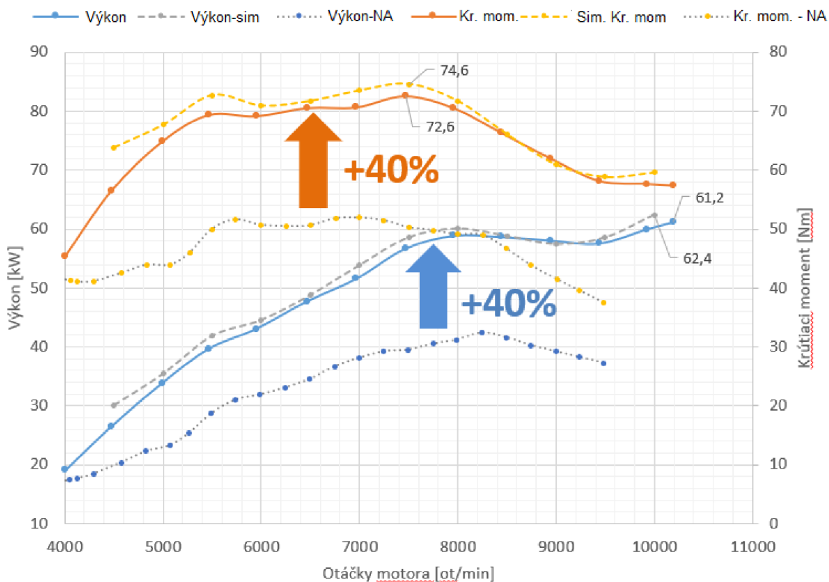
Obr. 13 Vonkajšia otáčková charakteristika motora monopostu Dragon – Porovnanie motora s prirodzeným sánim a turbodúchadlom [15]
