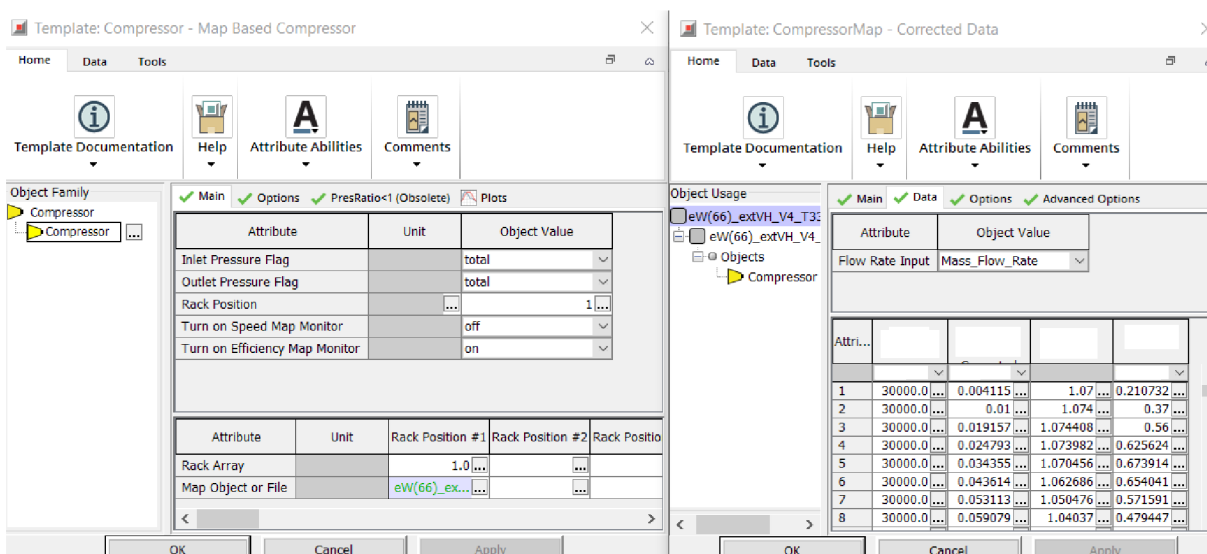
Obr. 38 Definícia kompresorovej mapy – E-compressor
