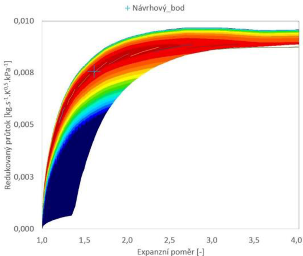
Obr. 12 Turbinová mapa s návrhovým pracovným bodom – NGT13[3]
