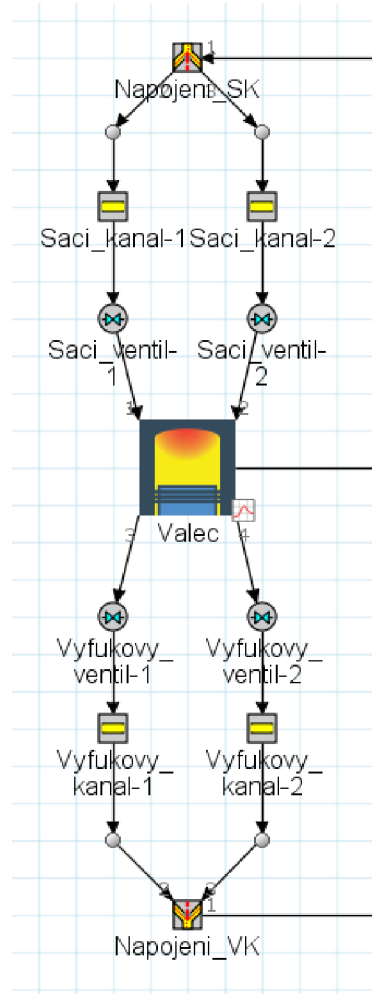
Obr. 20 Model valca a sacieho/vyfukového traktu
