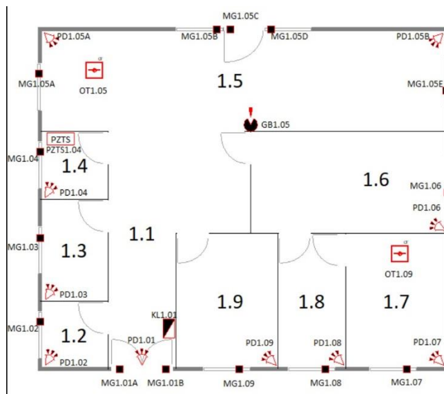
Obrázek 22 Modelový objekt
